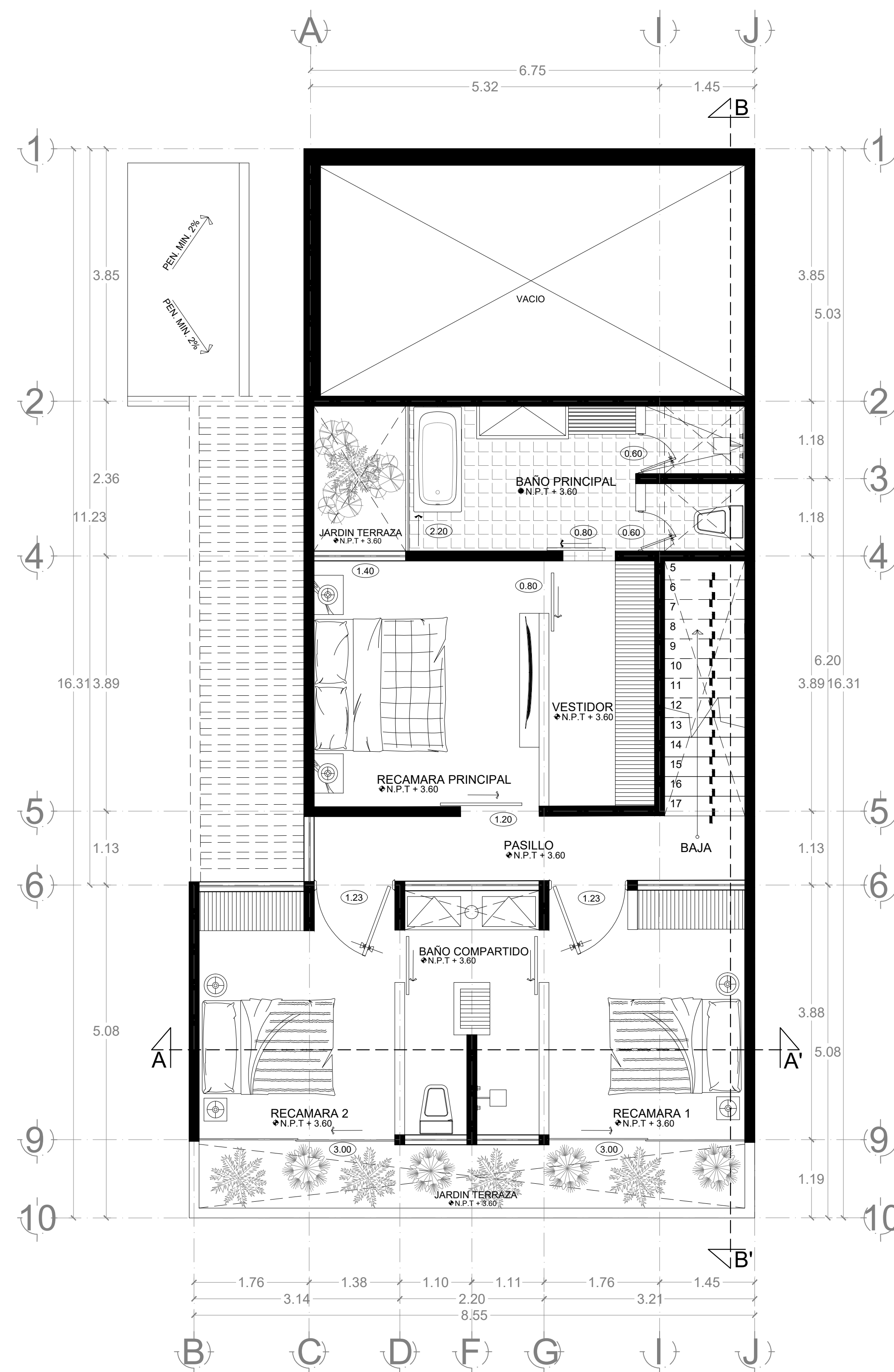
PLANTA ARQUITECTONICA ALTA ESC: 1:75
