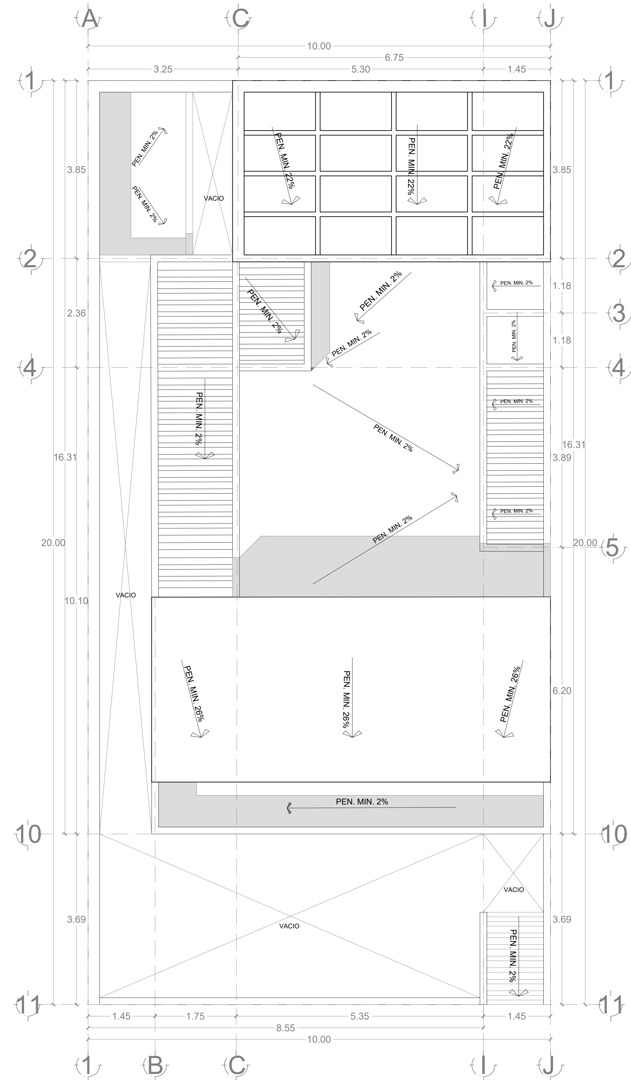
PLANTA ARQUITECTONICA DE CONJUNTO ESC: 1:75
