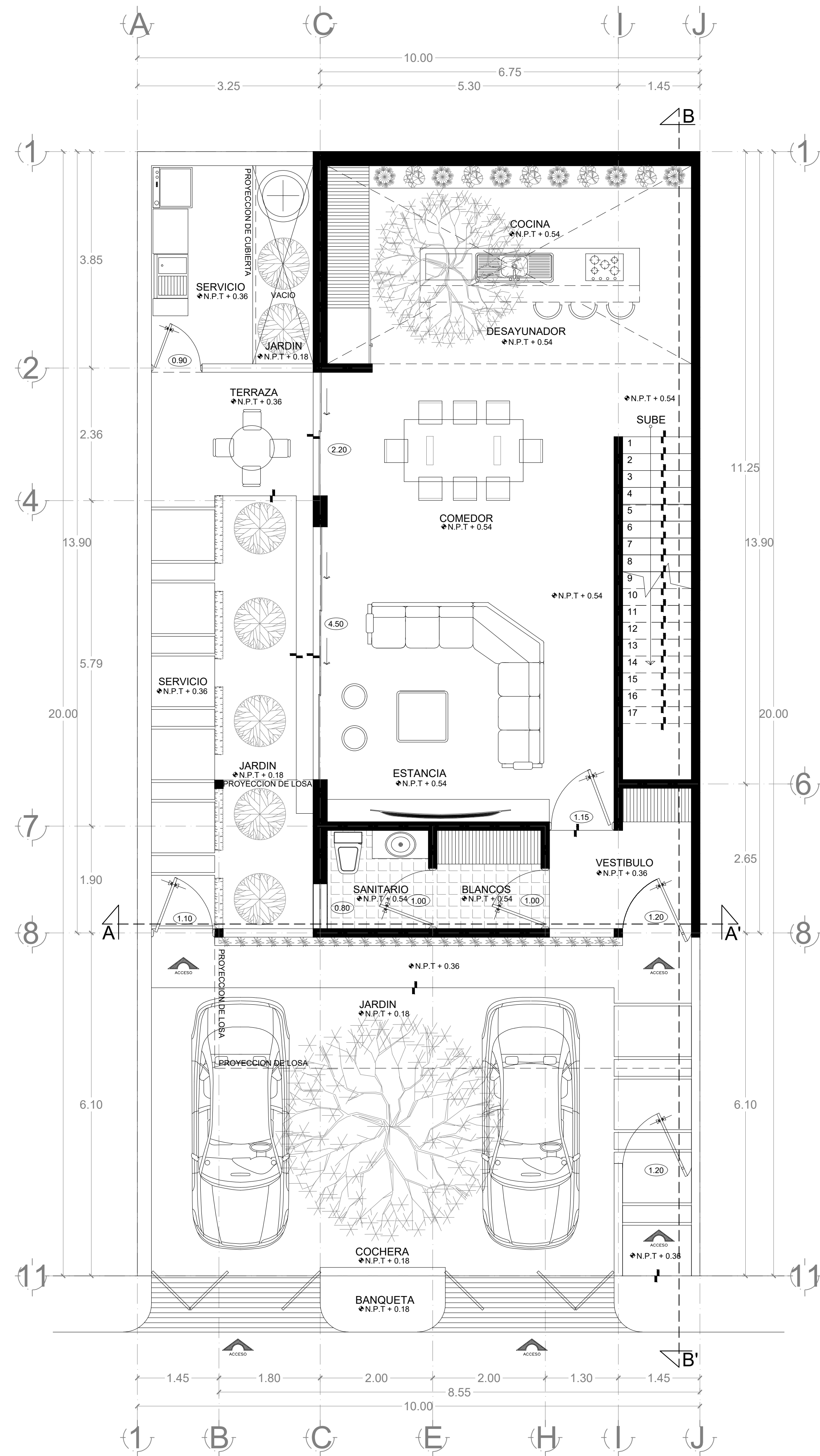
PLANTA ARQUITECTONICA BAJA ESC: 1:75
