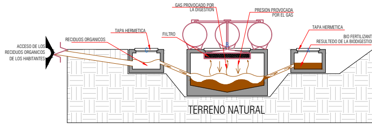
CORTE TRANSVERSAL A
