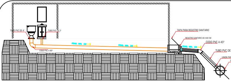
DIAGRAMA EN CORTE DE RECOLECCION A LA TOMA DE DRENAJE
