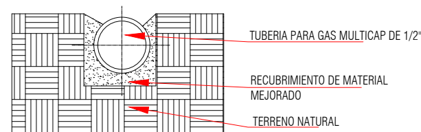
CORTE RECUBRIMIENTO MANGUERA
