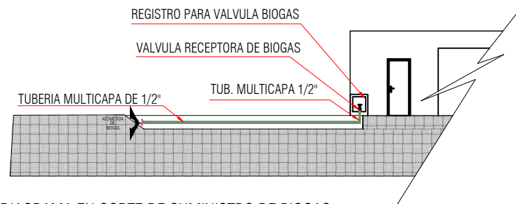
DIAGRAMA EN CORTE DE SUMINISTRO DE BIOGAS
