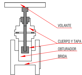
CORTE VALVULA DE GAS
