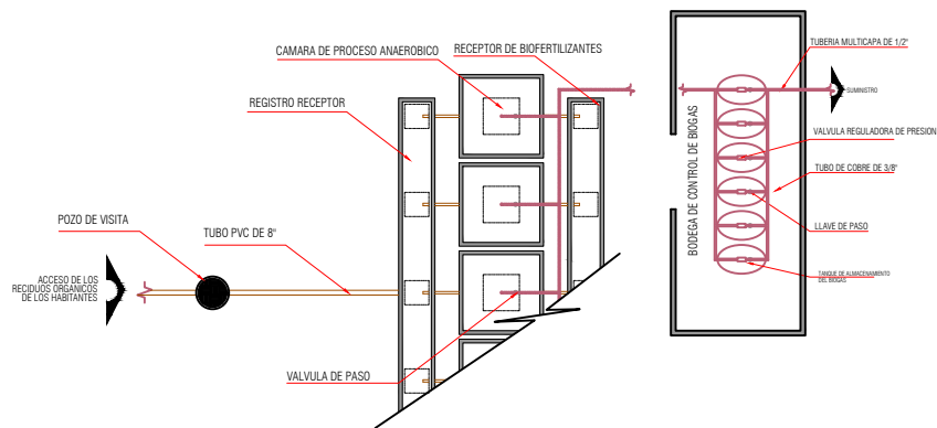
DIAGRAMA EN PLANTA DE PROCESO DE OBTENCION DEL BIOGAS
