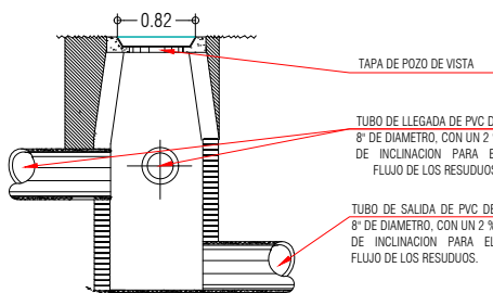
CORTE POZO DE VISTA
