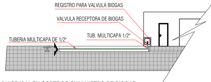
DIAGRAMA EN CORTE DE SUMINISTRO DE BIOGAS
