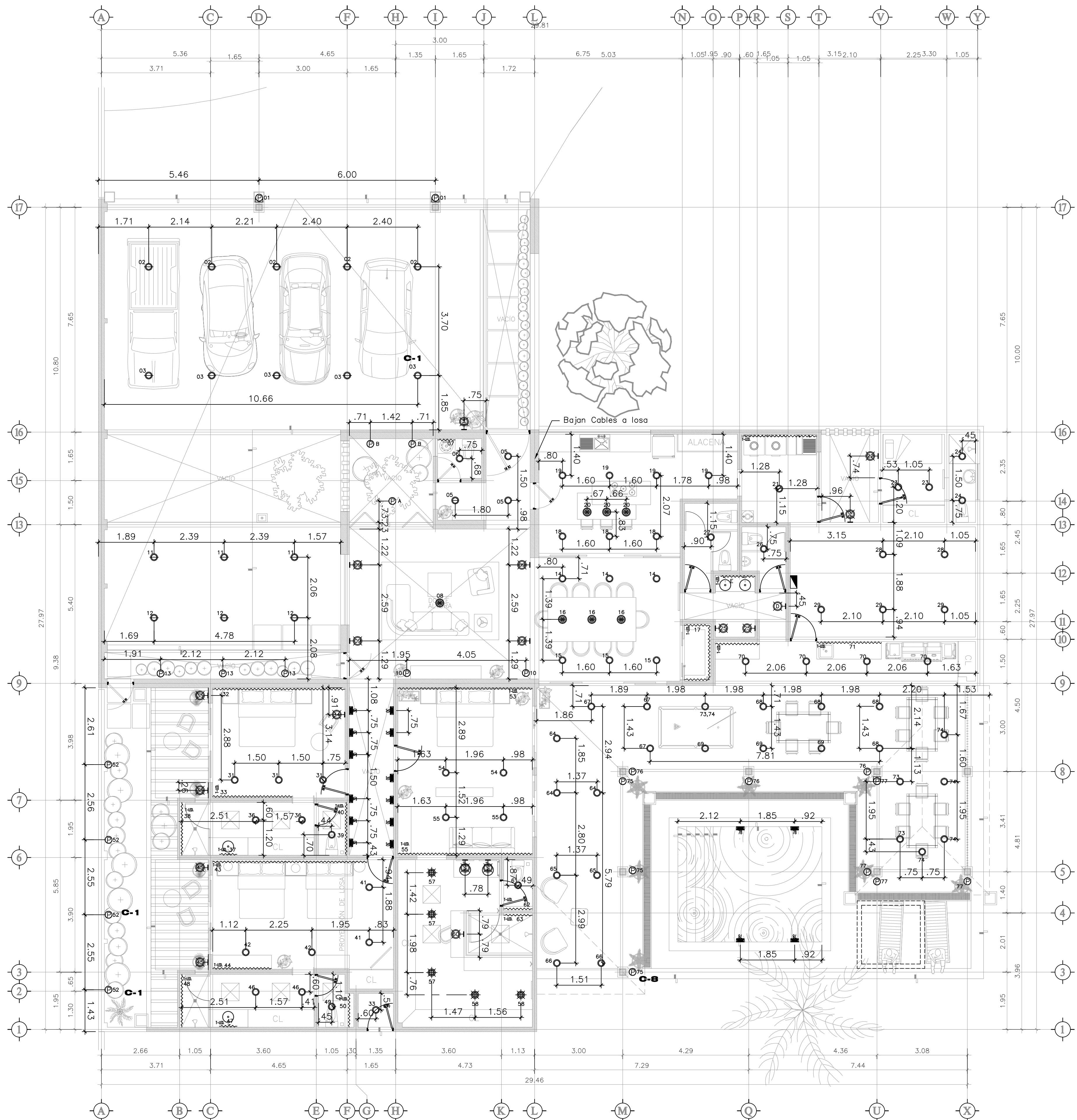
E 02 INSTALACION ELECTRICA - DISTANCIA DE LAMPARAS Escala: ..... 1/75 Acot.: ..... MIL
