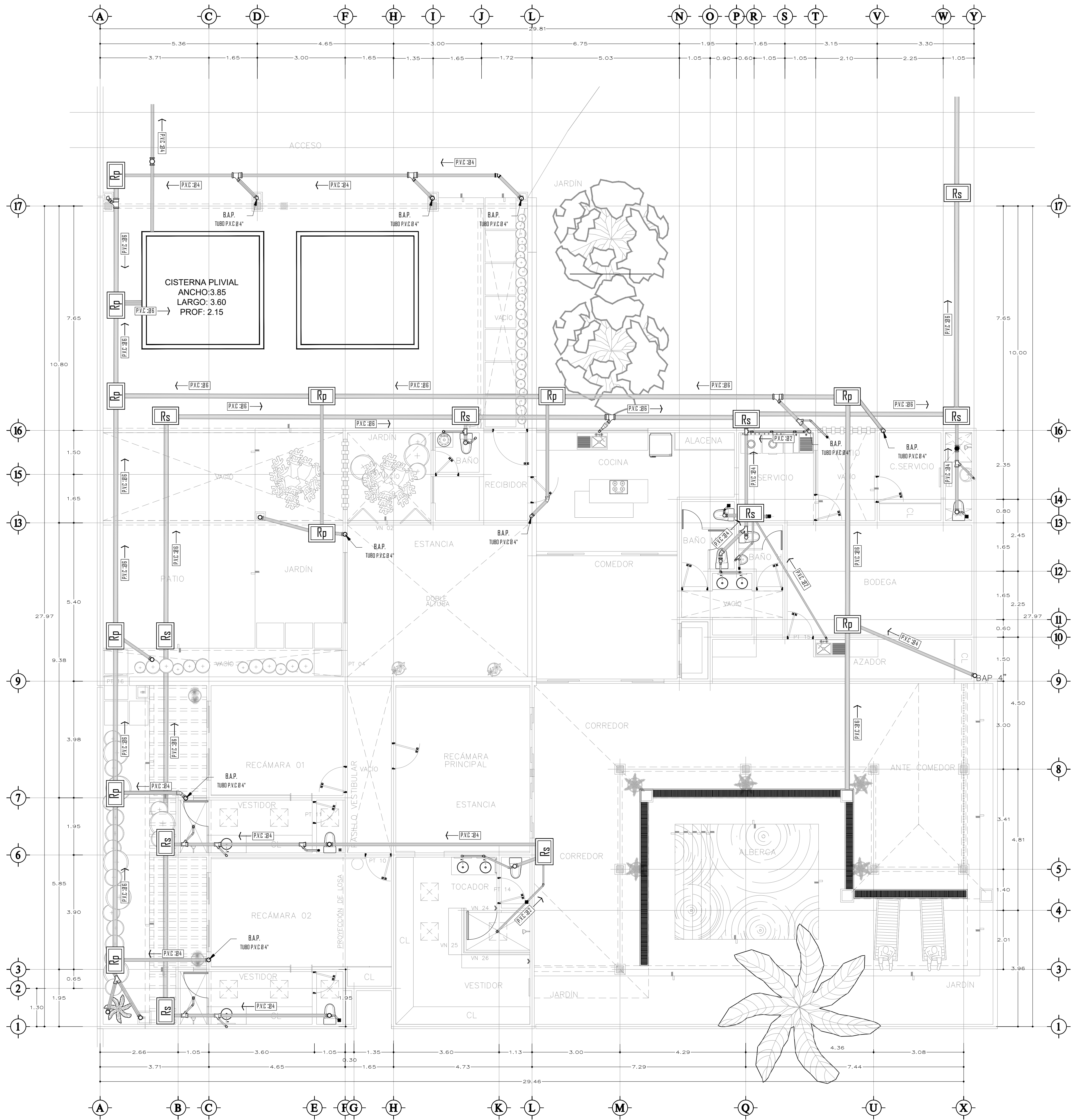
IS 01 PLANTA ARQUITECTONICA - INSTALACION SANITARIA
