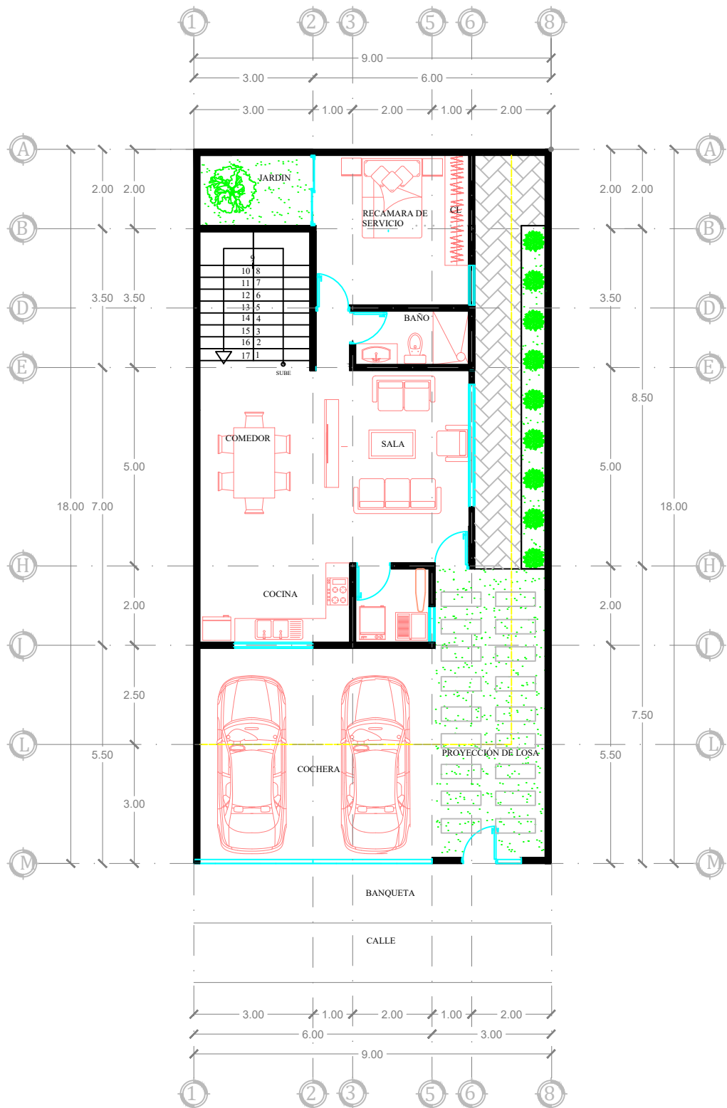
PLANTA BAJA
