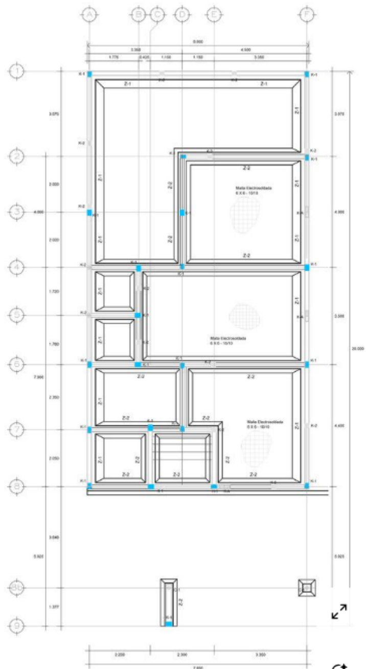
PLANTA DE CIMENTACION Esc. 1:100 Aoot. mts.
