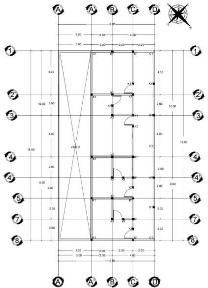
PLANTA ALTA ESC: 1:50
