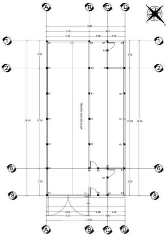
PLANTA BAJA ESC: 1:50
