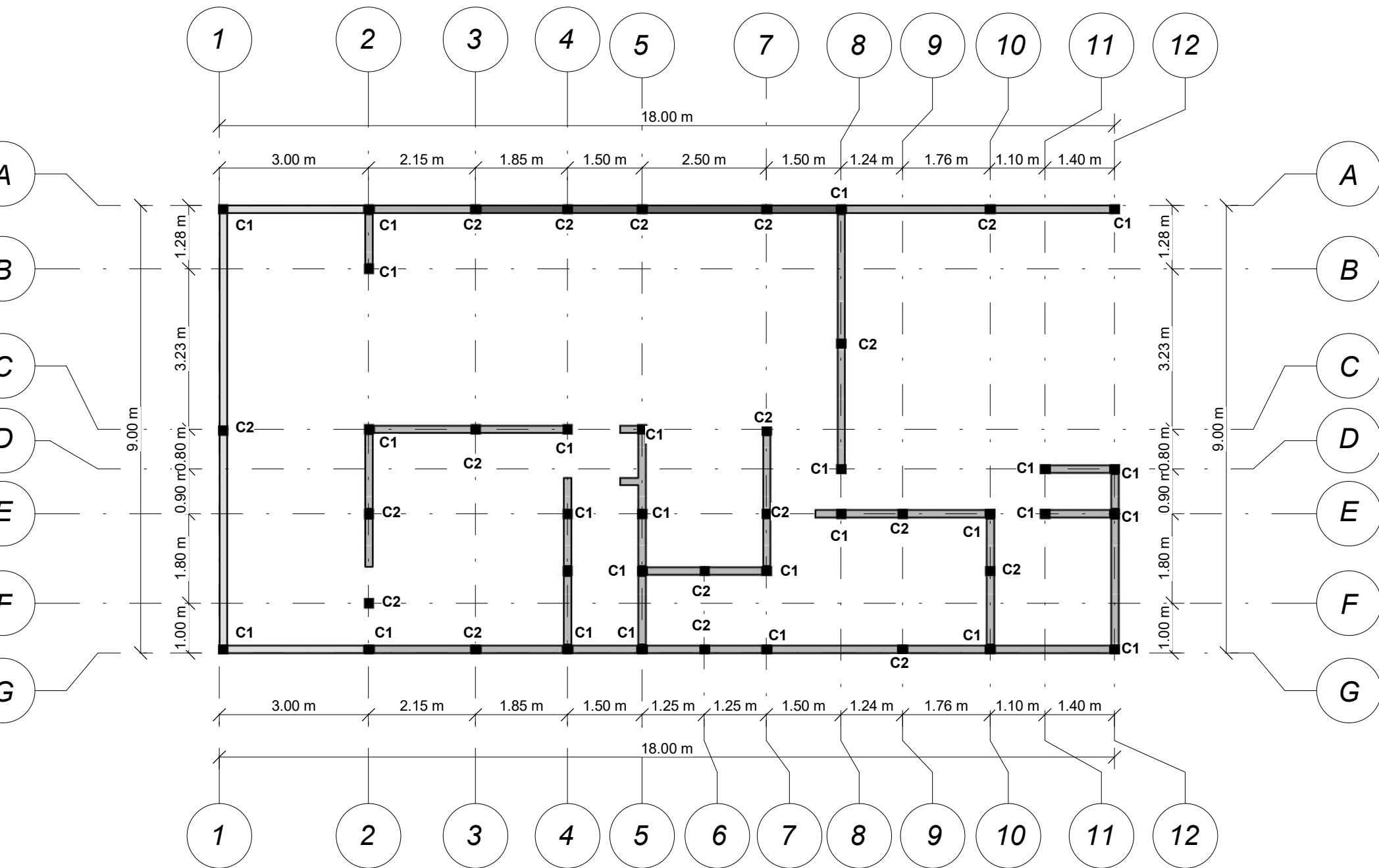
PLANTA ARQUITECTONICA ESTRUCTURAL
