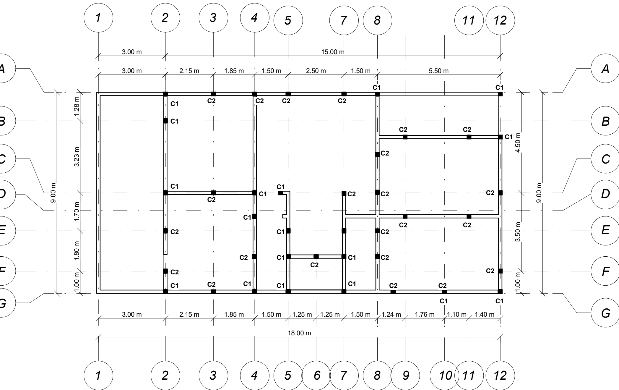
PLANTA ARQUITECTONICA ESTRUCTURAL PLANTA ALTA
