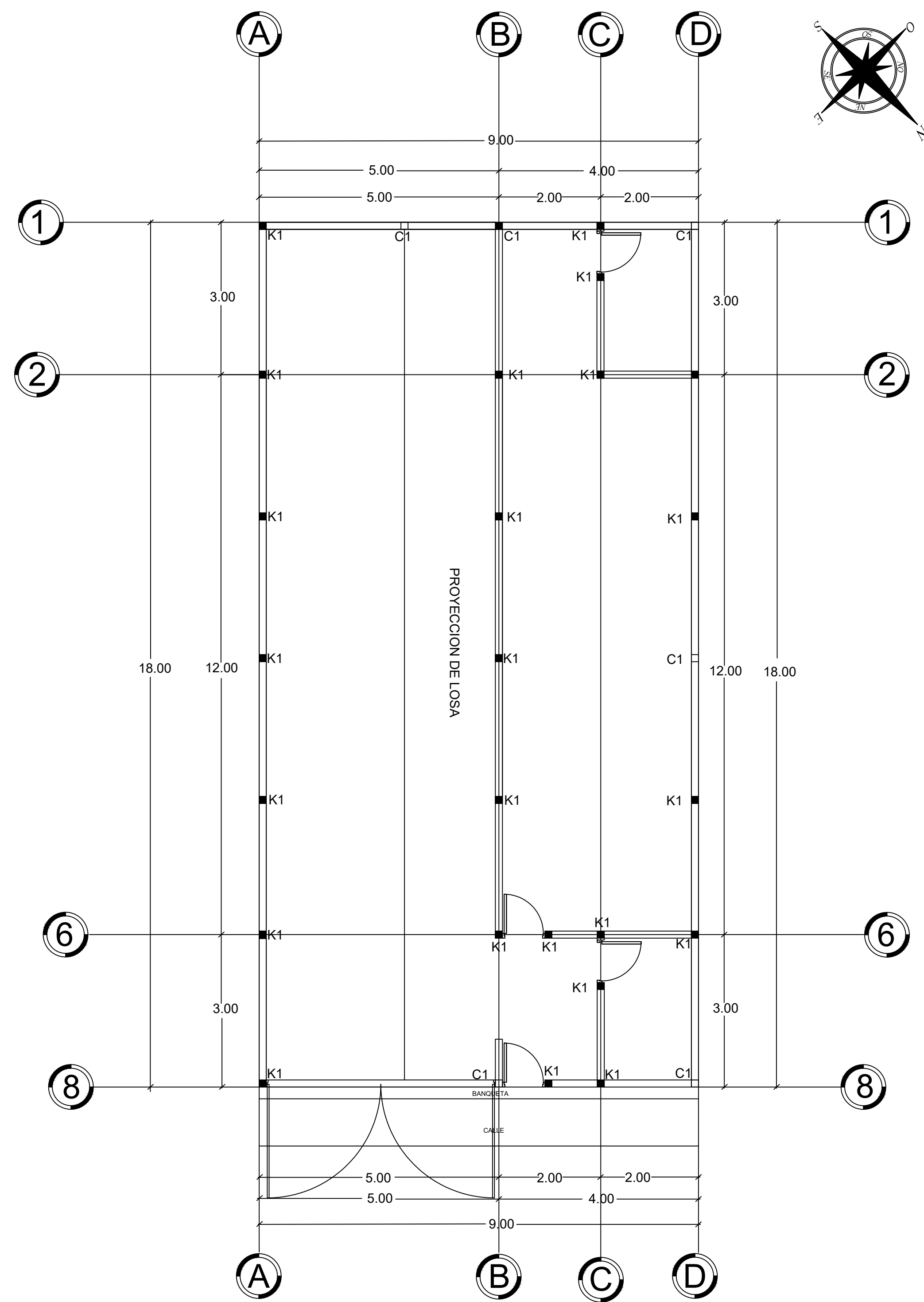
PLANTA BAJA ESC: 1:50
