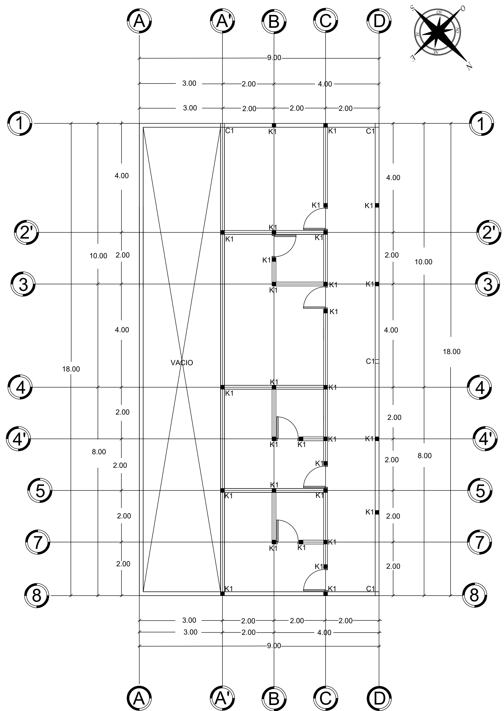
PLANTA ALTA ESC: 1:50
