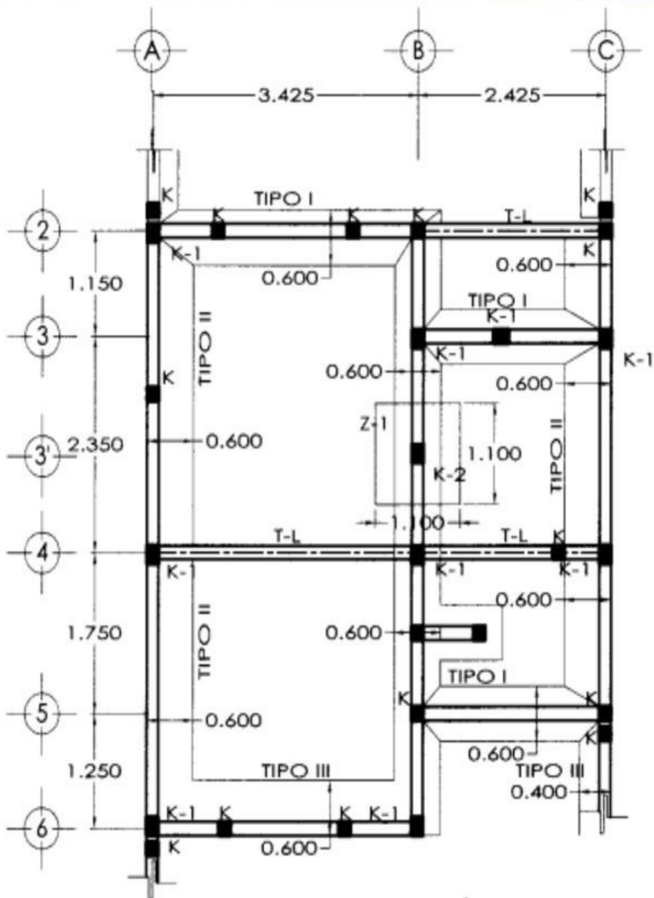
PLANTA DE CIMENTACIÓN
