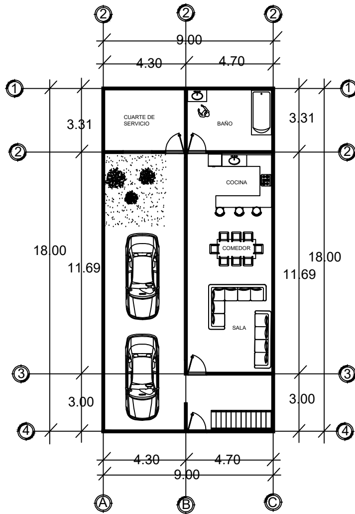
PLANTA BAJA ESC: 1:50
