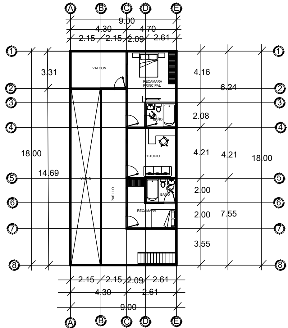
PLANTA ALTA ESC: 1:50
