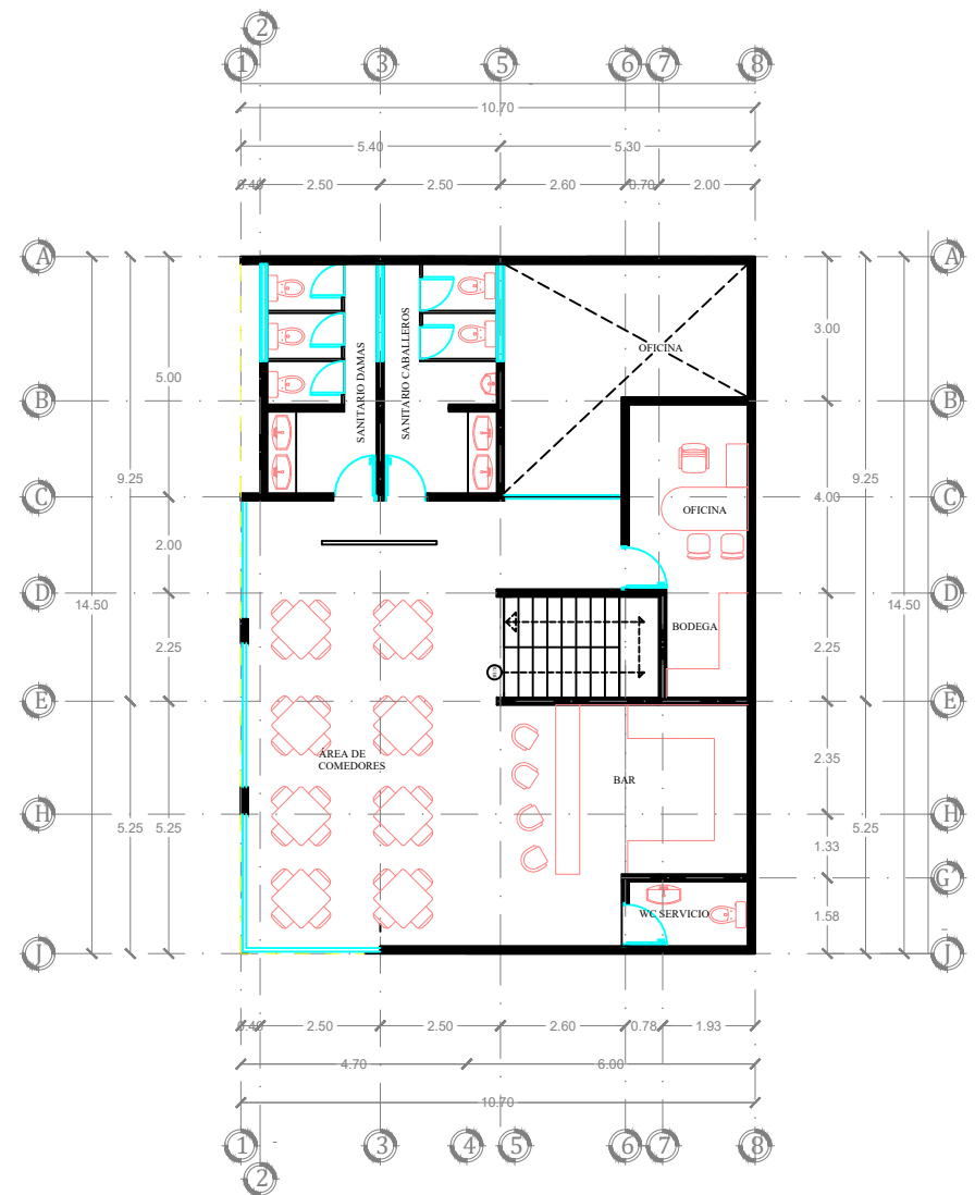
PLANTA ALTA ESC: 1:50
