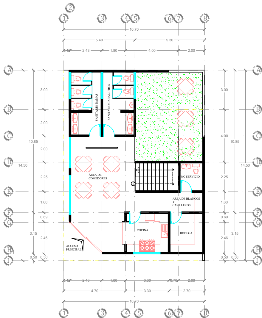
PLANTA BAJA ESC: 1:50
