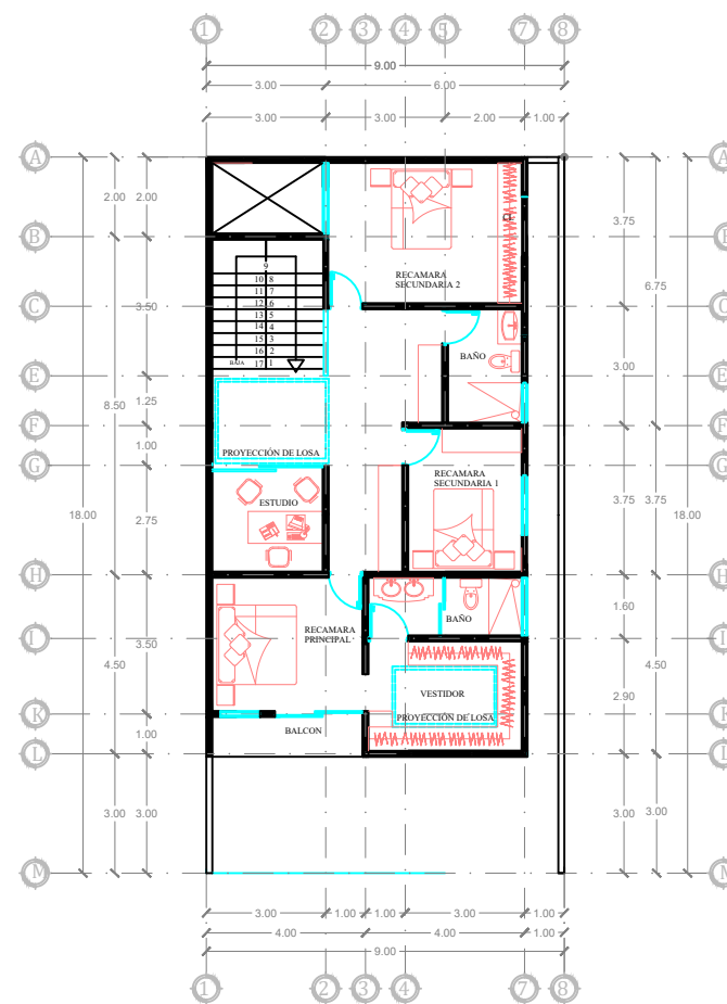
PLANTA ALTA
