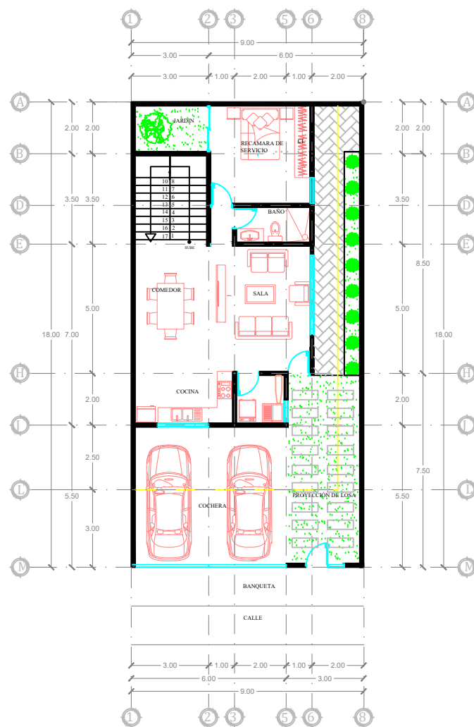
PLANTA BAJA
