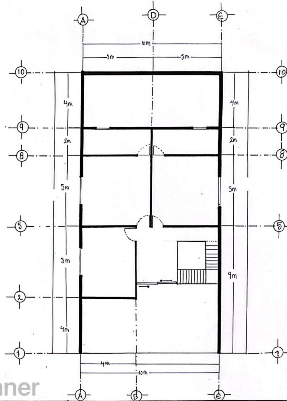
Primer nivel.
