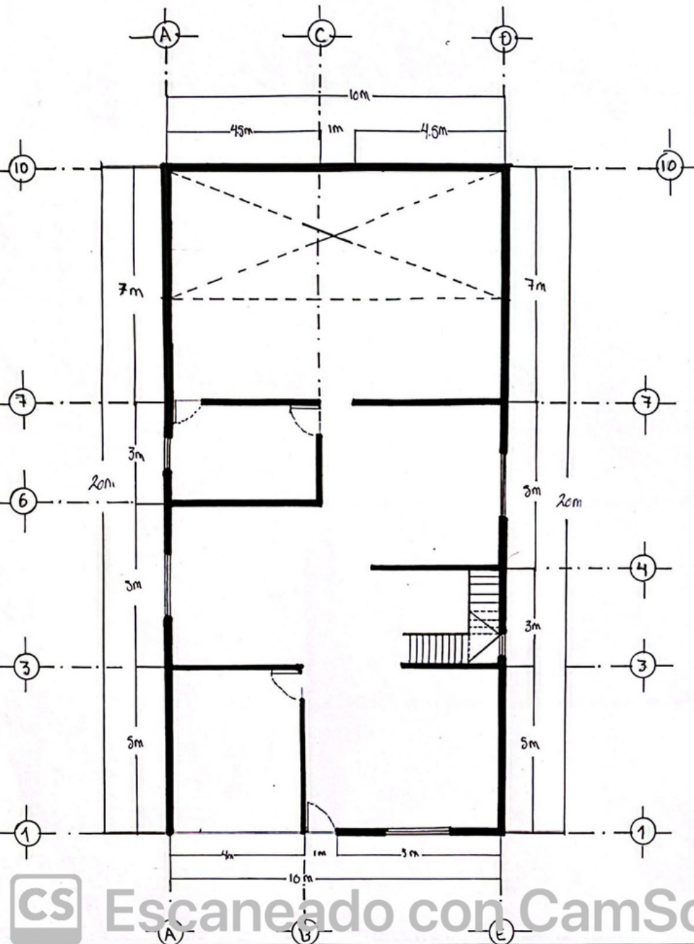
Planta baja
