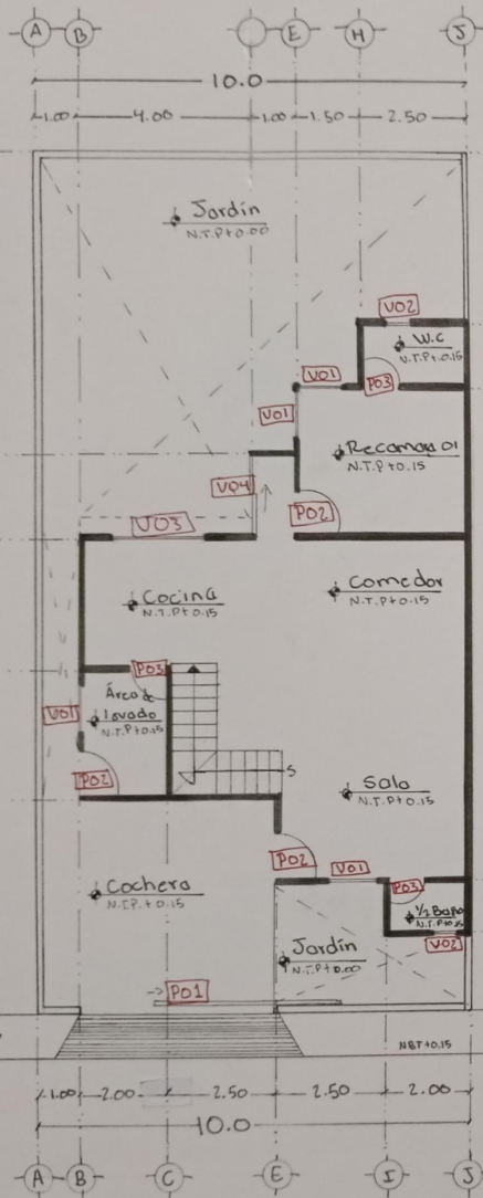
Planta Arquitectonica Baja.
