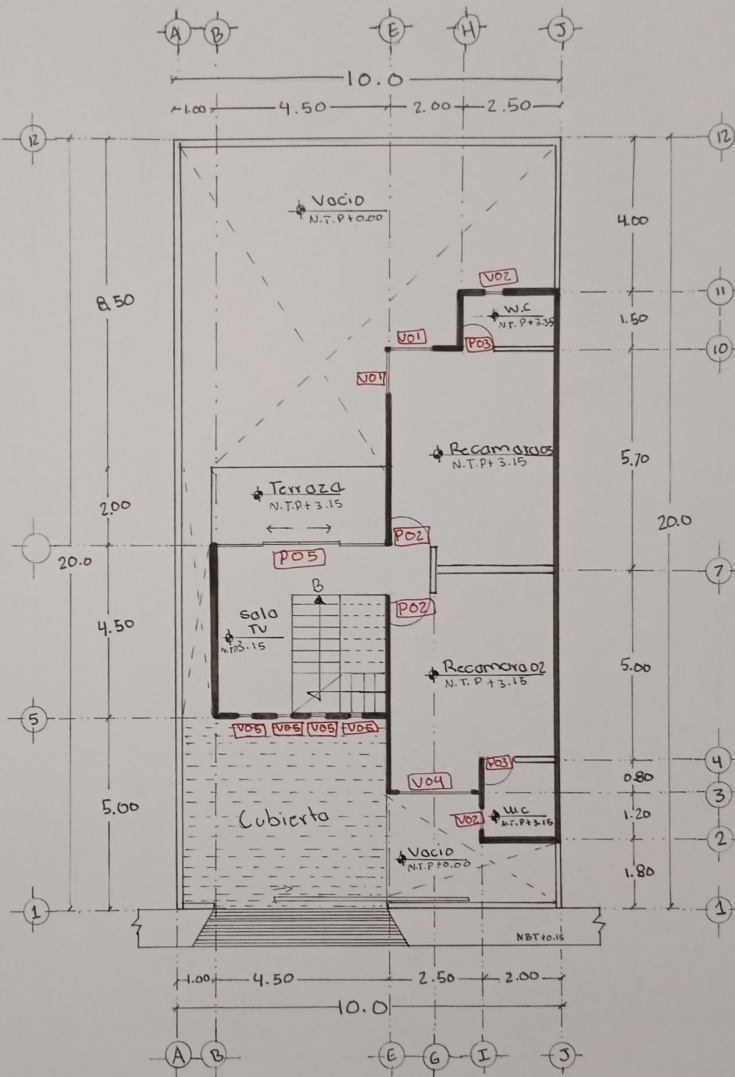
Planta Arquitectonica Primer Nivel.
