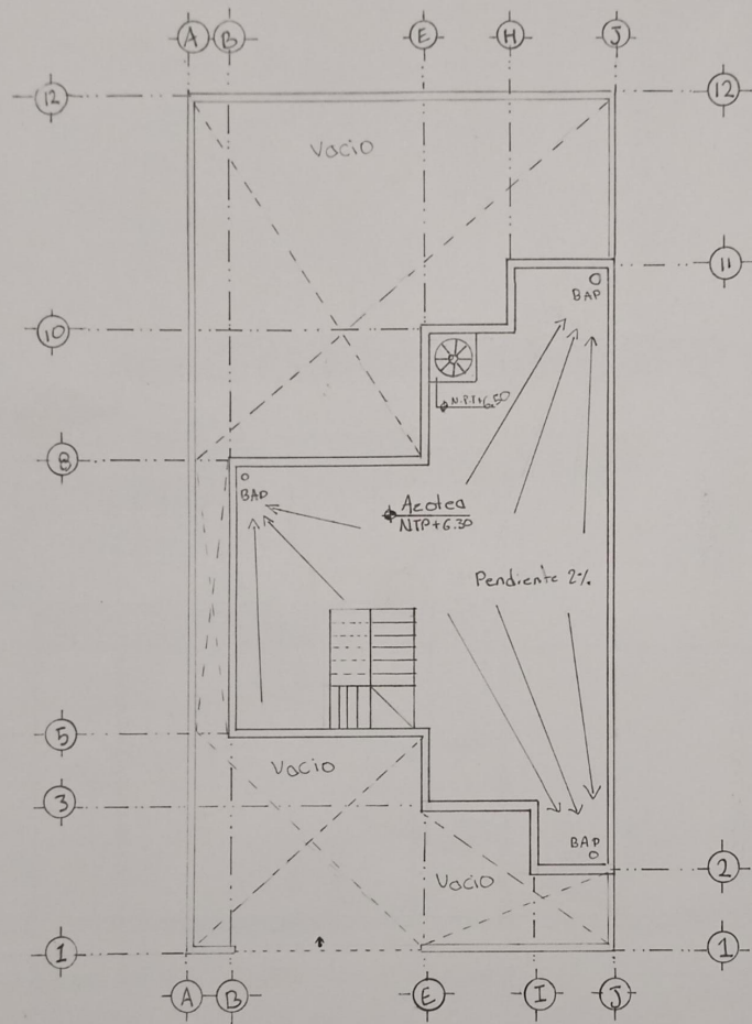
Planta de Azotea
