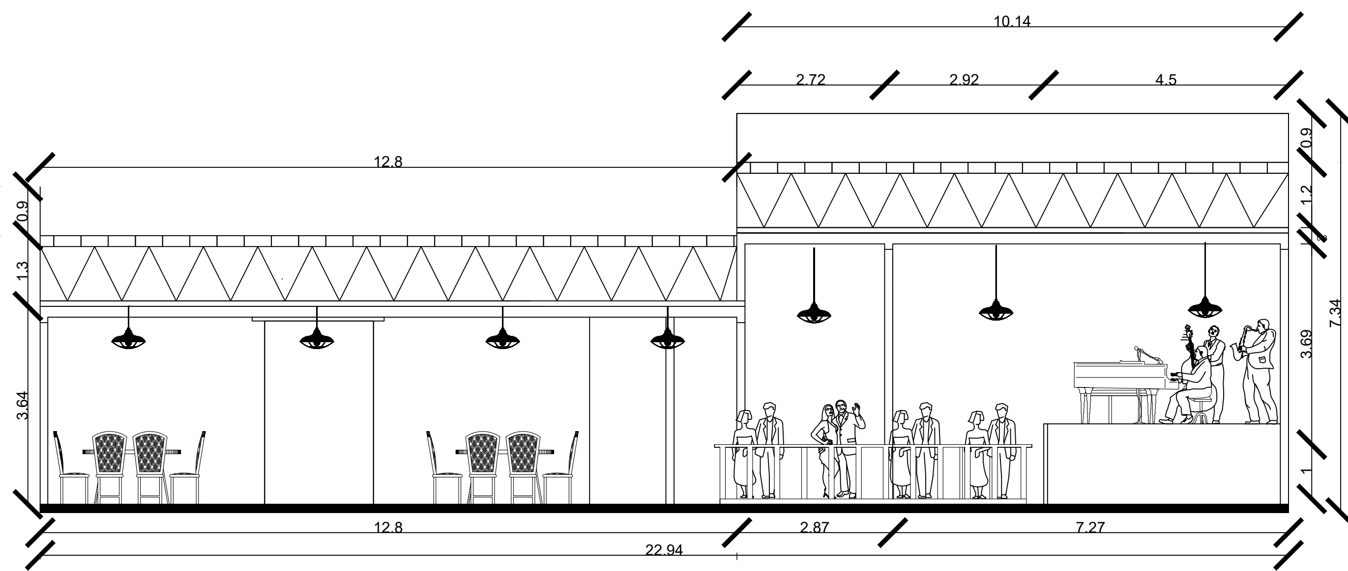
CORTE TRANSVERSAL A - A'
