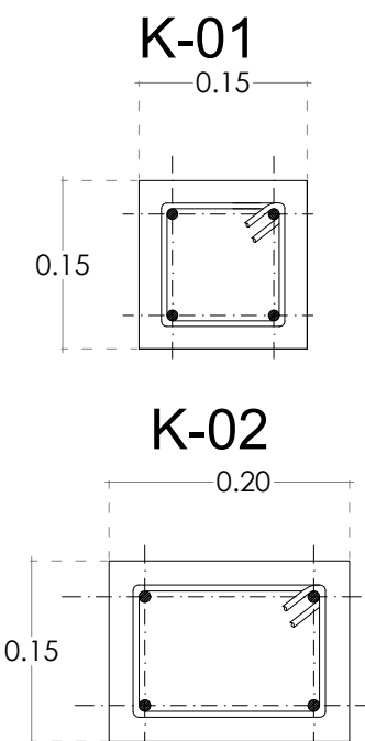
CASTILLO DE 0.15 X 0.15 M. ARMADA CON 4 VARILLA DE \frac{3}{8} " ESTRIBOS @ 15 CMS DE VARILLA DE NO. 2, COLADA CON CONCRETO 150 KG/CM2
