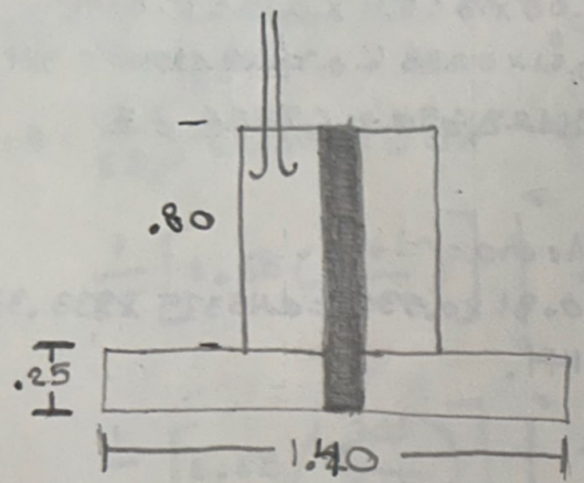
Zapata ejemplo columnas
