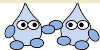
cohesion
