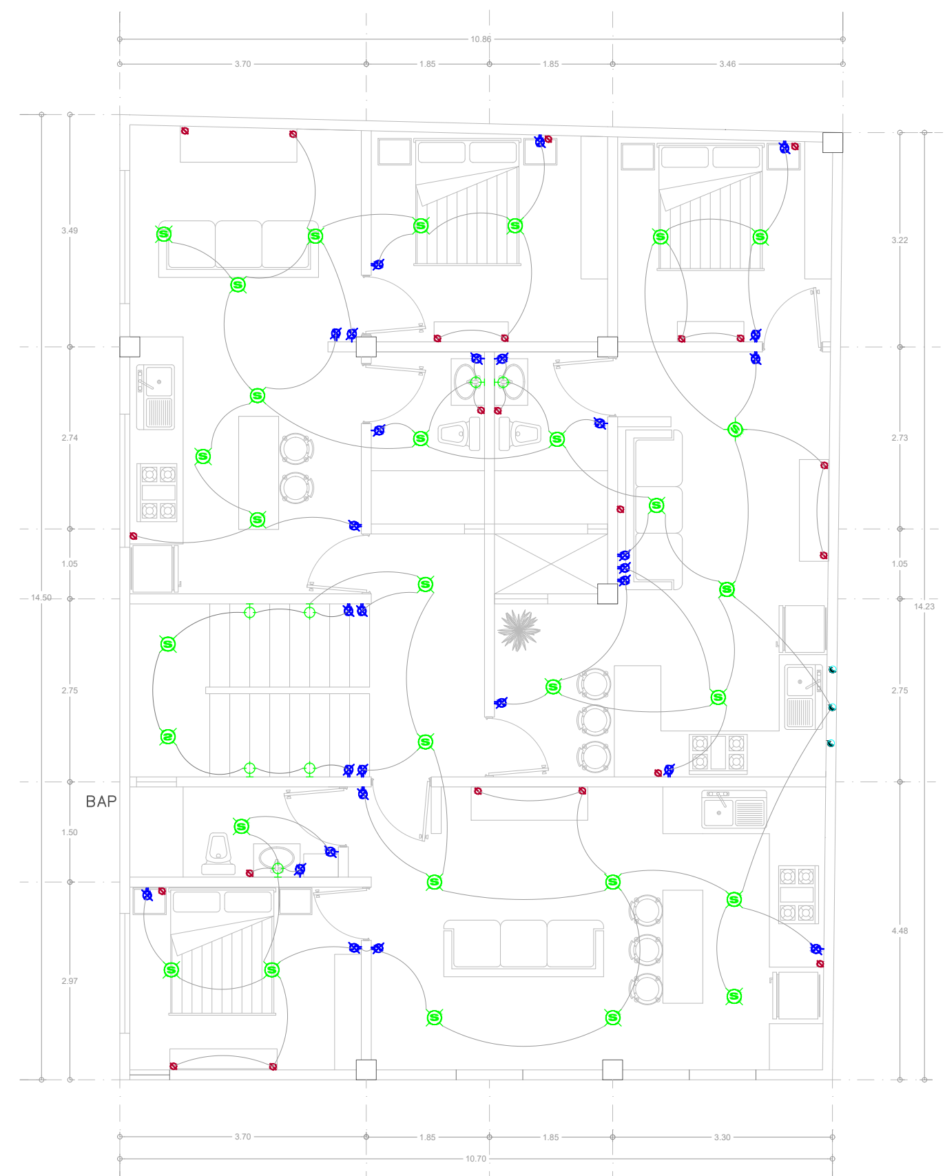
TERCERA PLANTA
