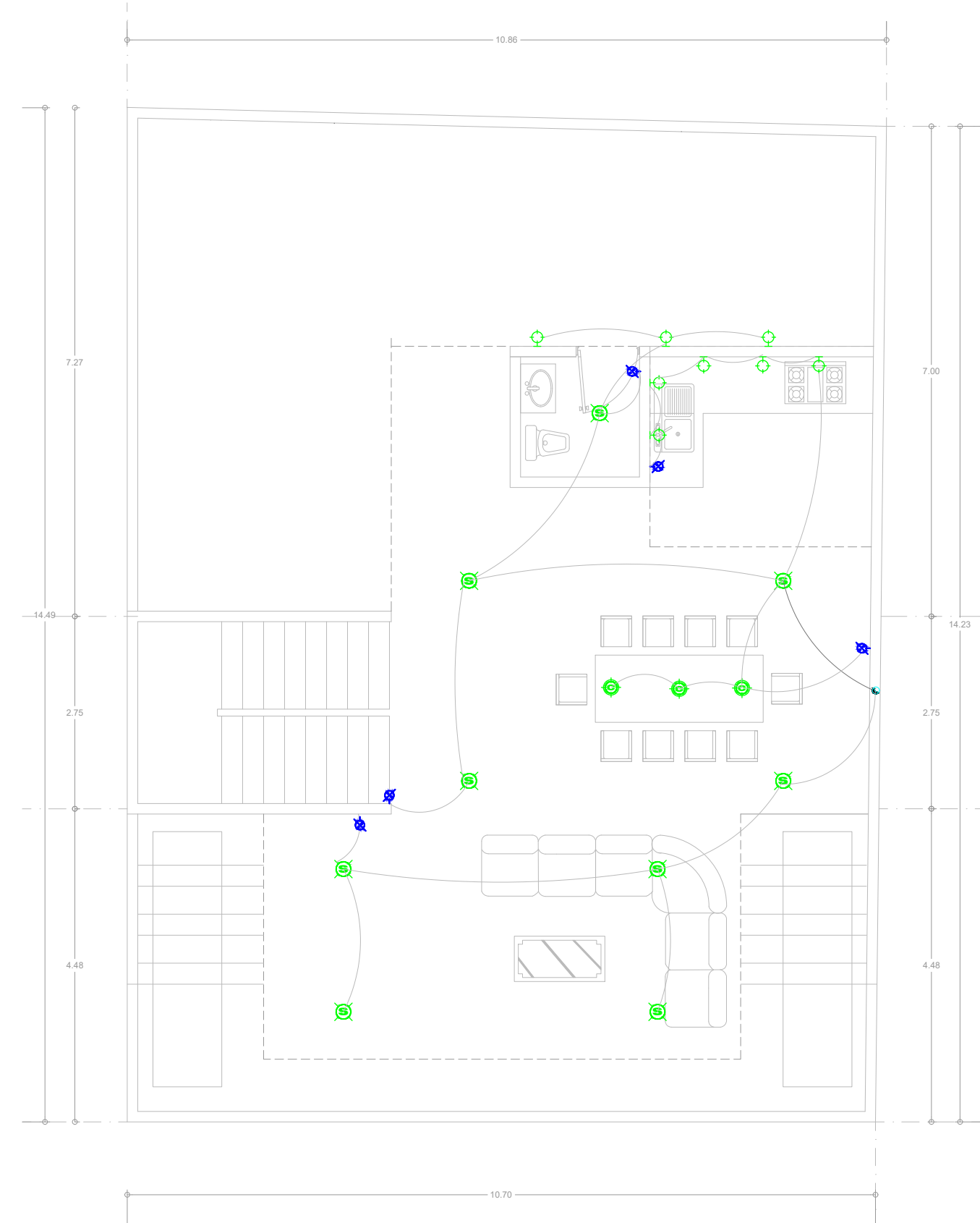
PLANTA AZOTEA
