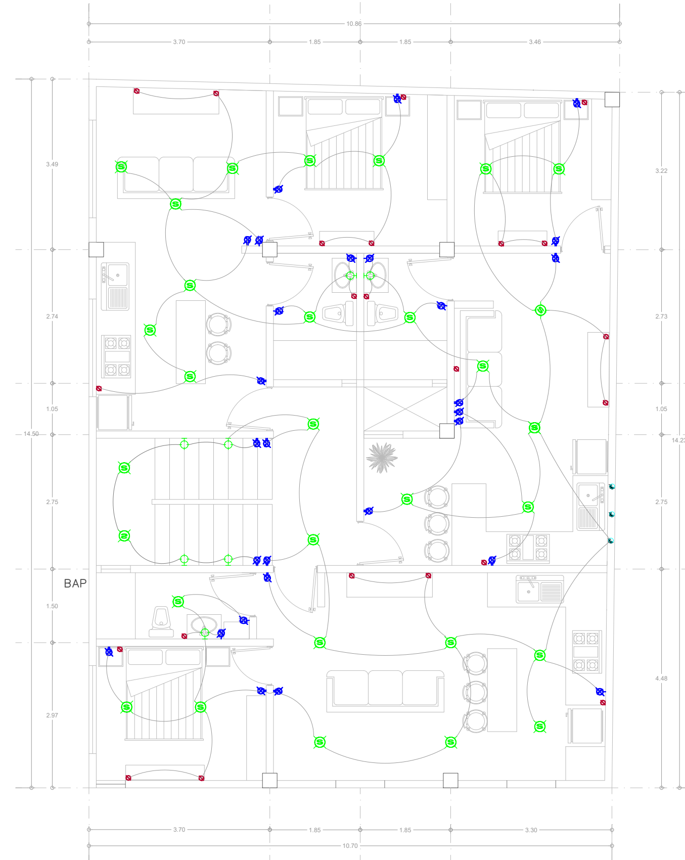
SEGUNDA PLANTA
