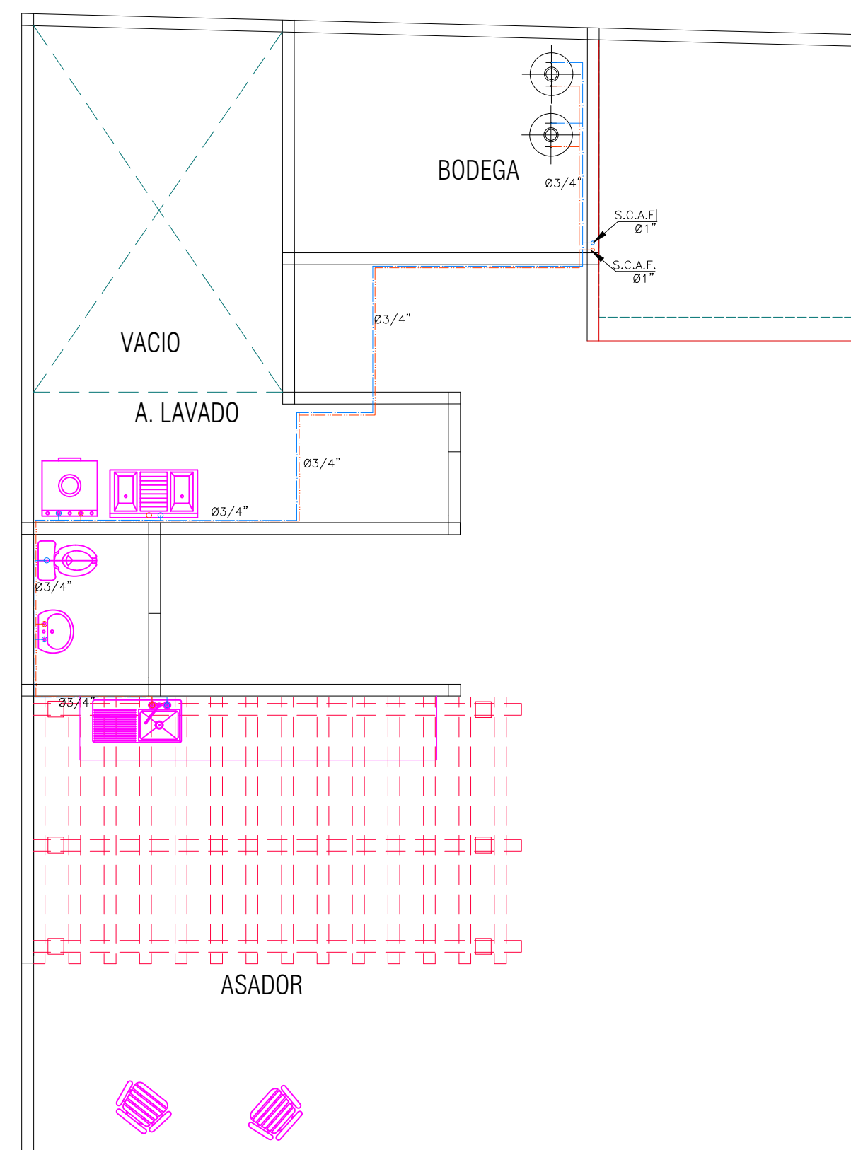
CUARTA PLANTA
