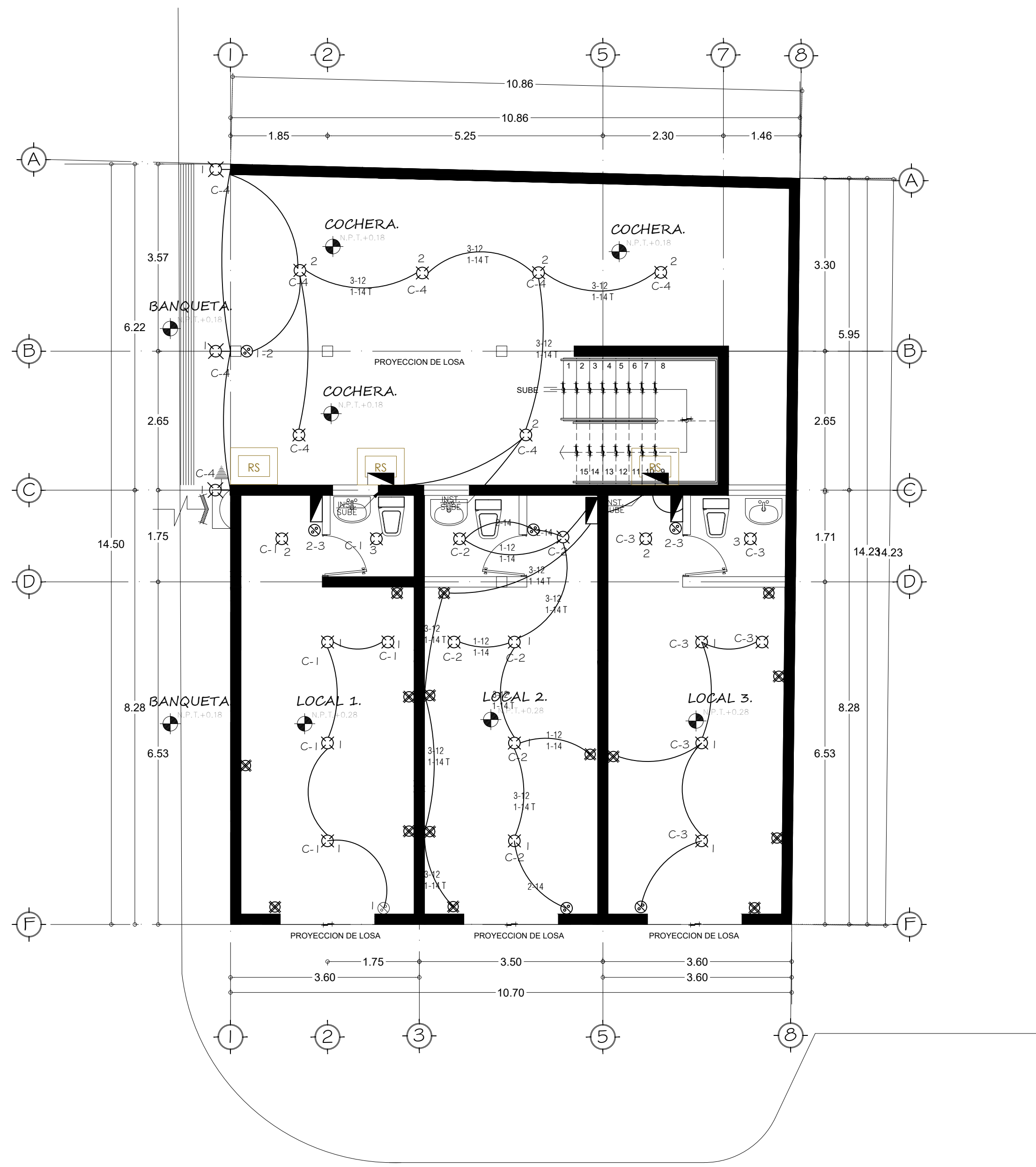
1 PLANTA BAJA
