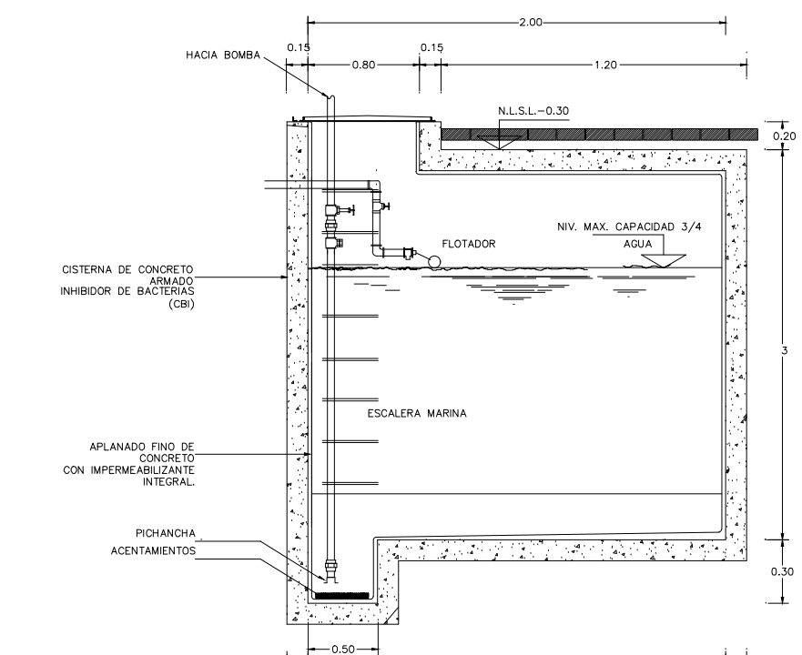
DETALLE DE CISTERNA SIN ESC
