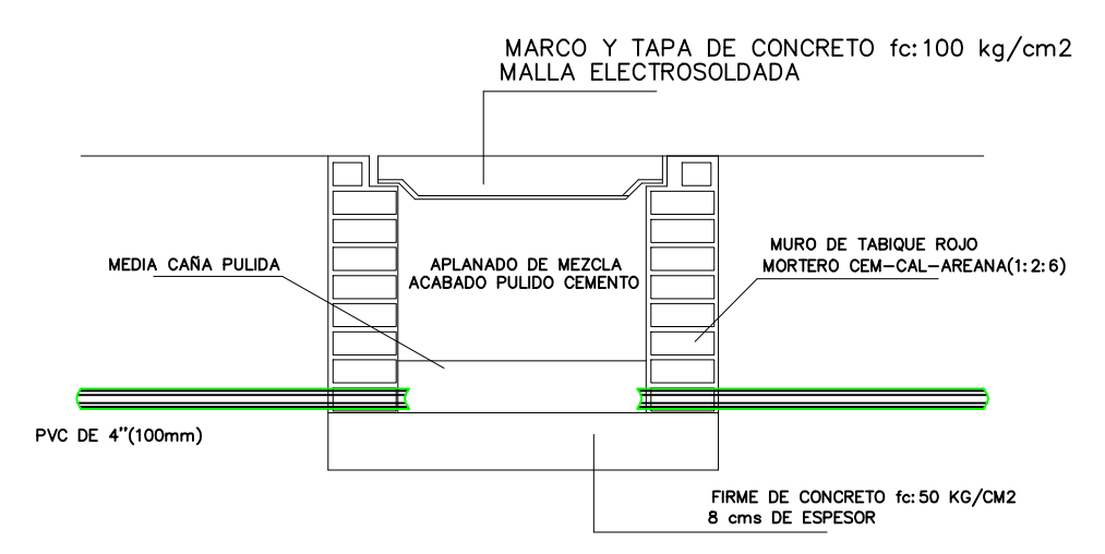
DETALLE DE REGISTRO SANITARIO Y PLUVIAL
