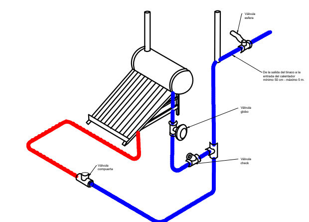
DETALLE DE CALENTADOR SIN ESC
