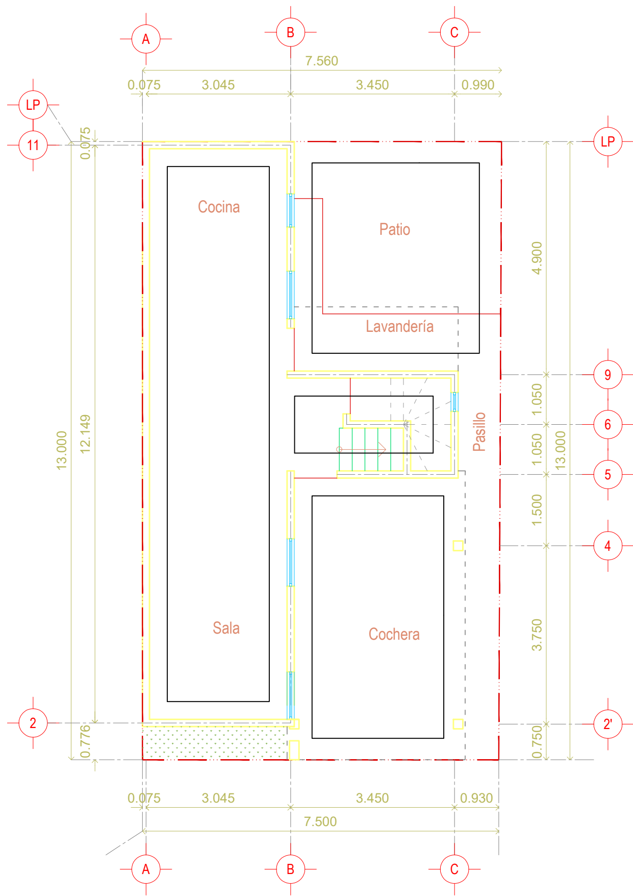
PLANTA BAJA
