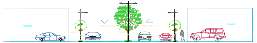
CORTE DE LA CALLE PRINCIPAL
