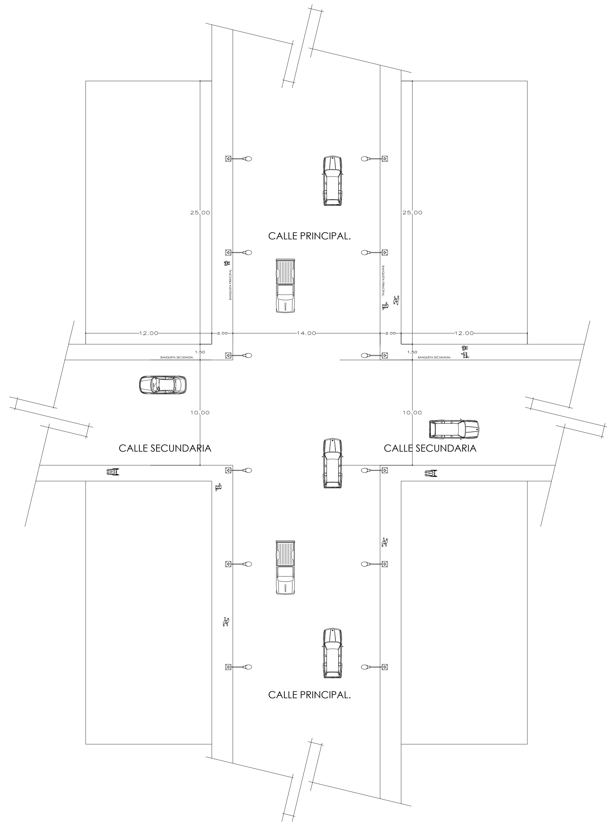
ARQ 01 TIPO RESIDENCIAL Escala _____ Acot. _____ Mts.
