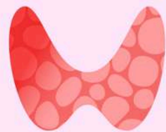
Tiroiditis
