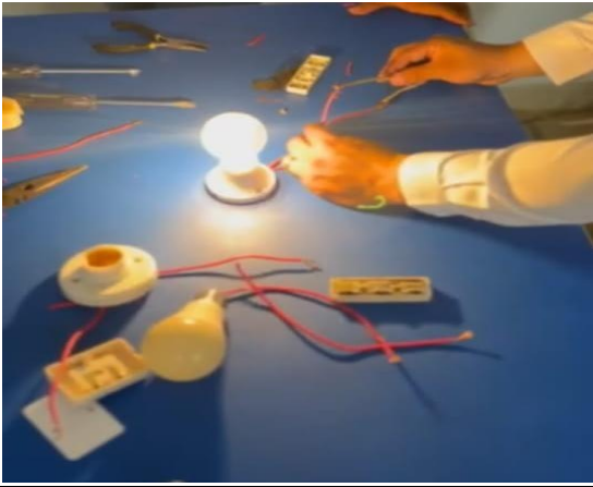
Se realizo un circuito en paralelo con 2 focos.
