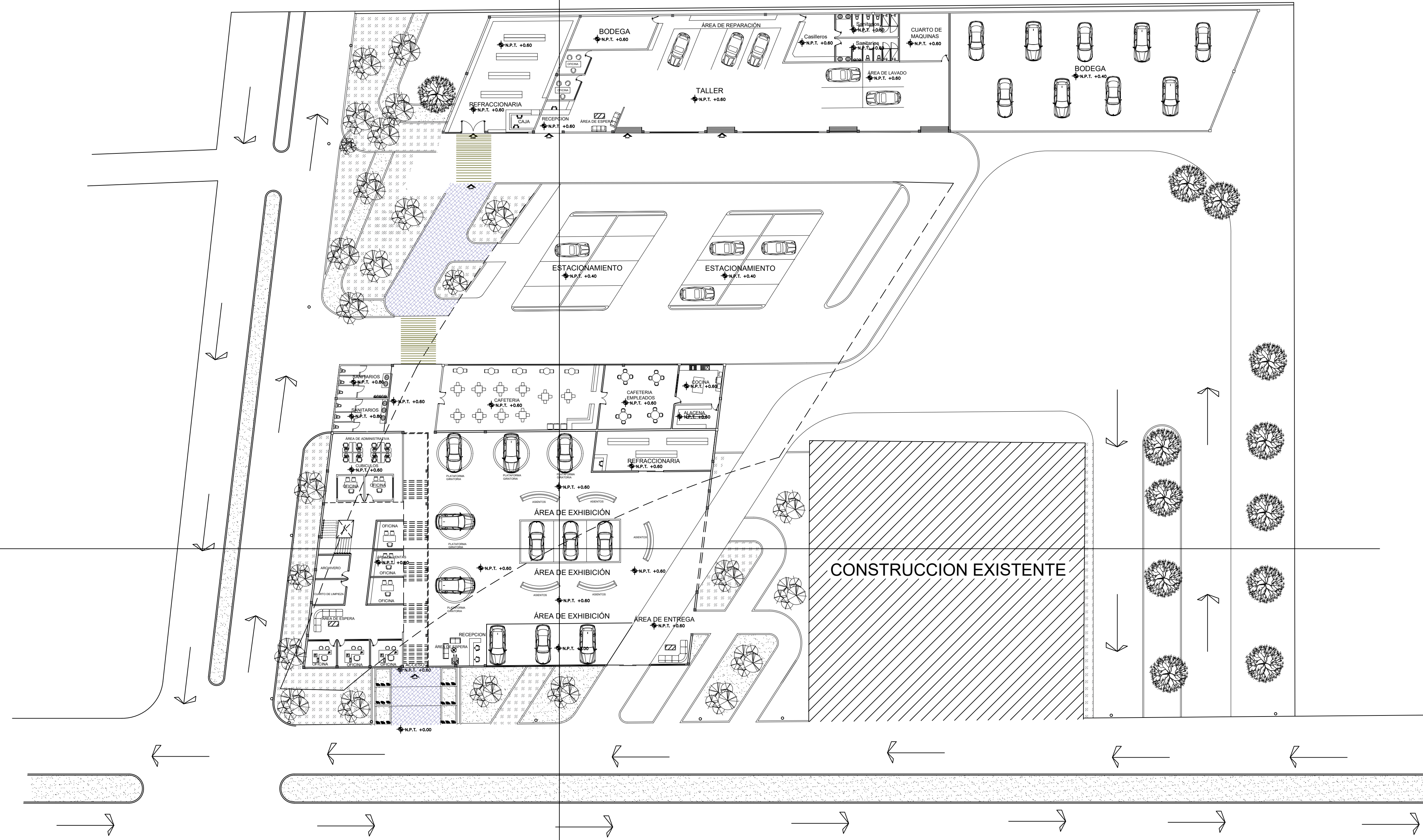
PLANTA ARQUITECTÓNICA BAJA ESC..... 1:400
