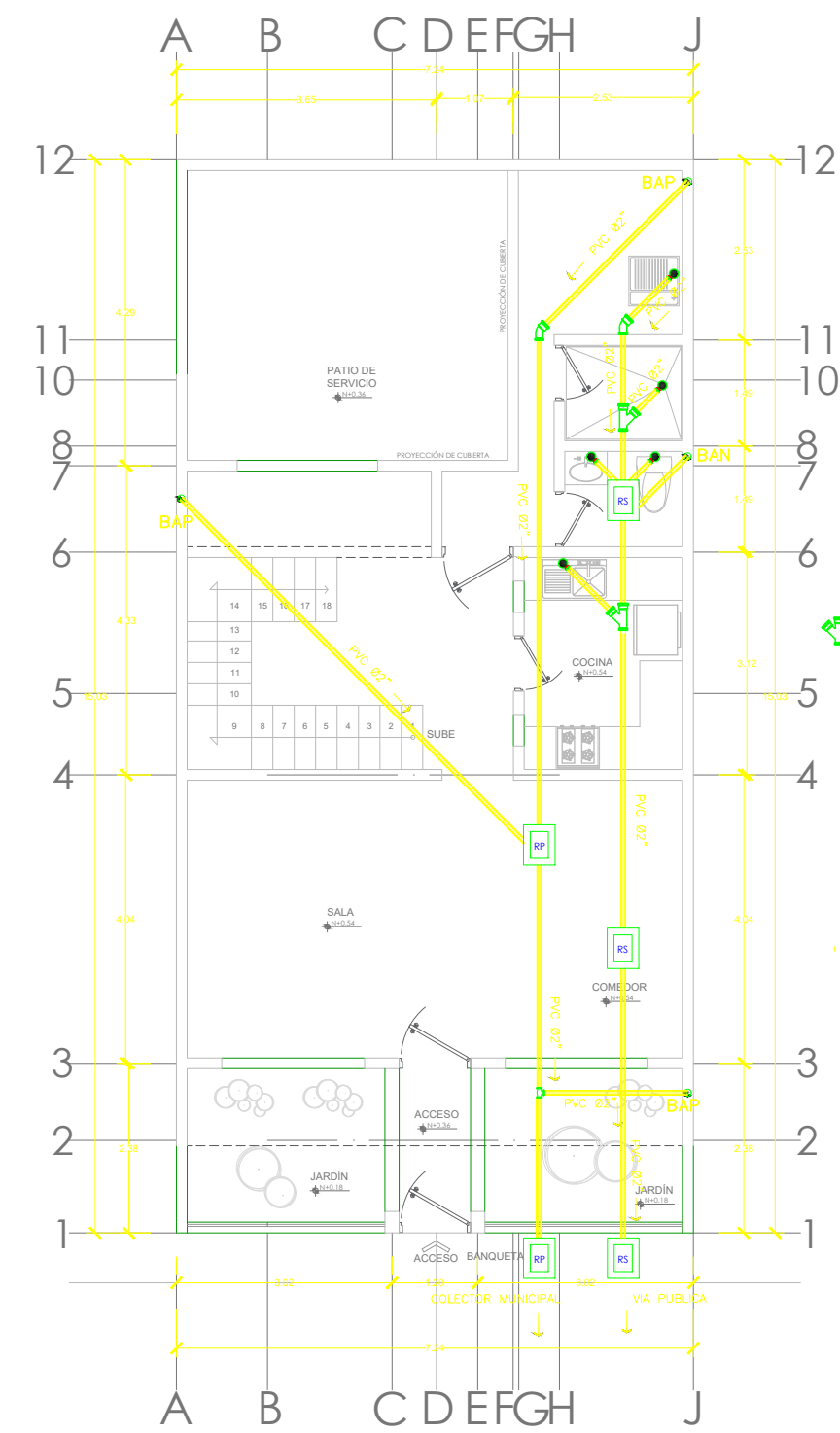
Planta Arquitectónica Baja
