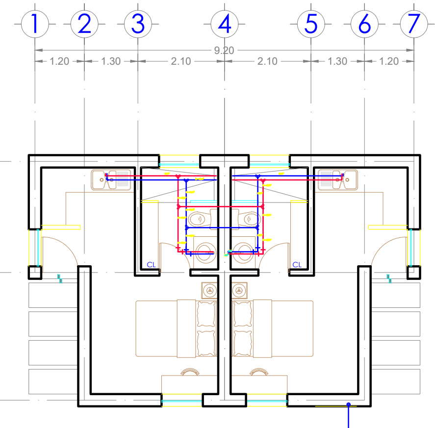
Planta Arquitectónica Única Estudiantiles 01
