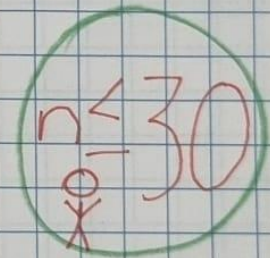
Pruebas estadísticas
