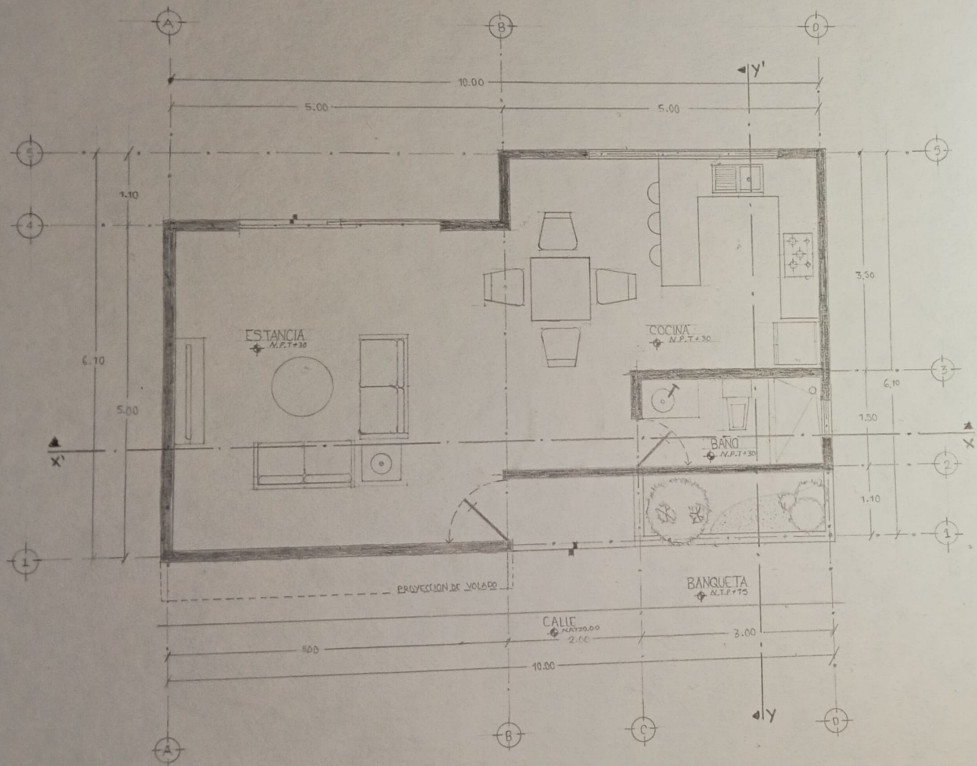
PLANTA ARQUITECTONICA ESC. 1:5 ACOT. M
