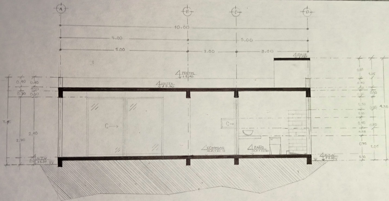
CORTE TRANSVERSAL X-X' ACOT...M ESC...1:50
