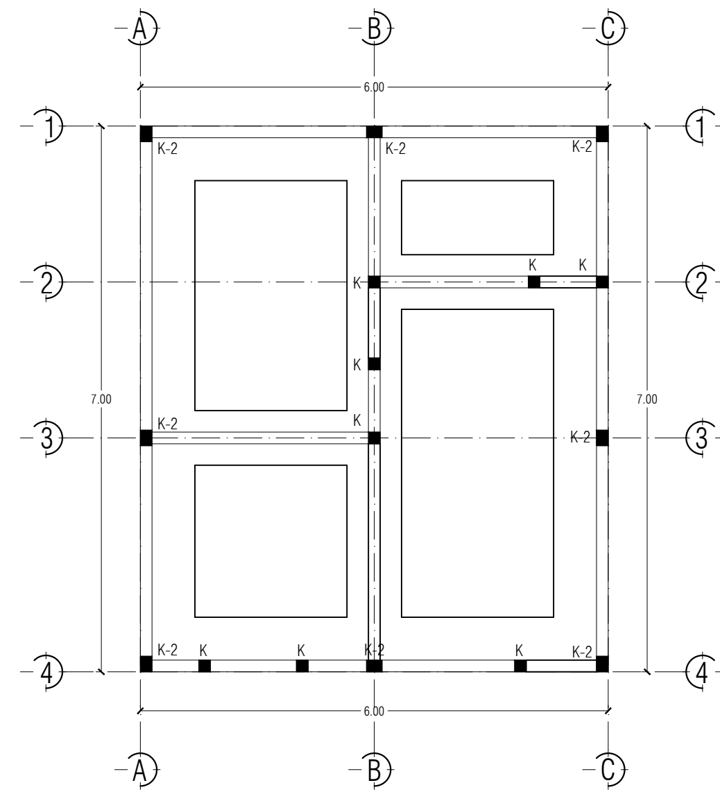
PLANTA DE CIMENTACIÓN
