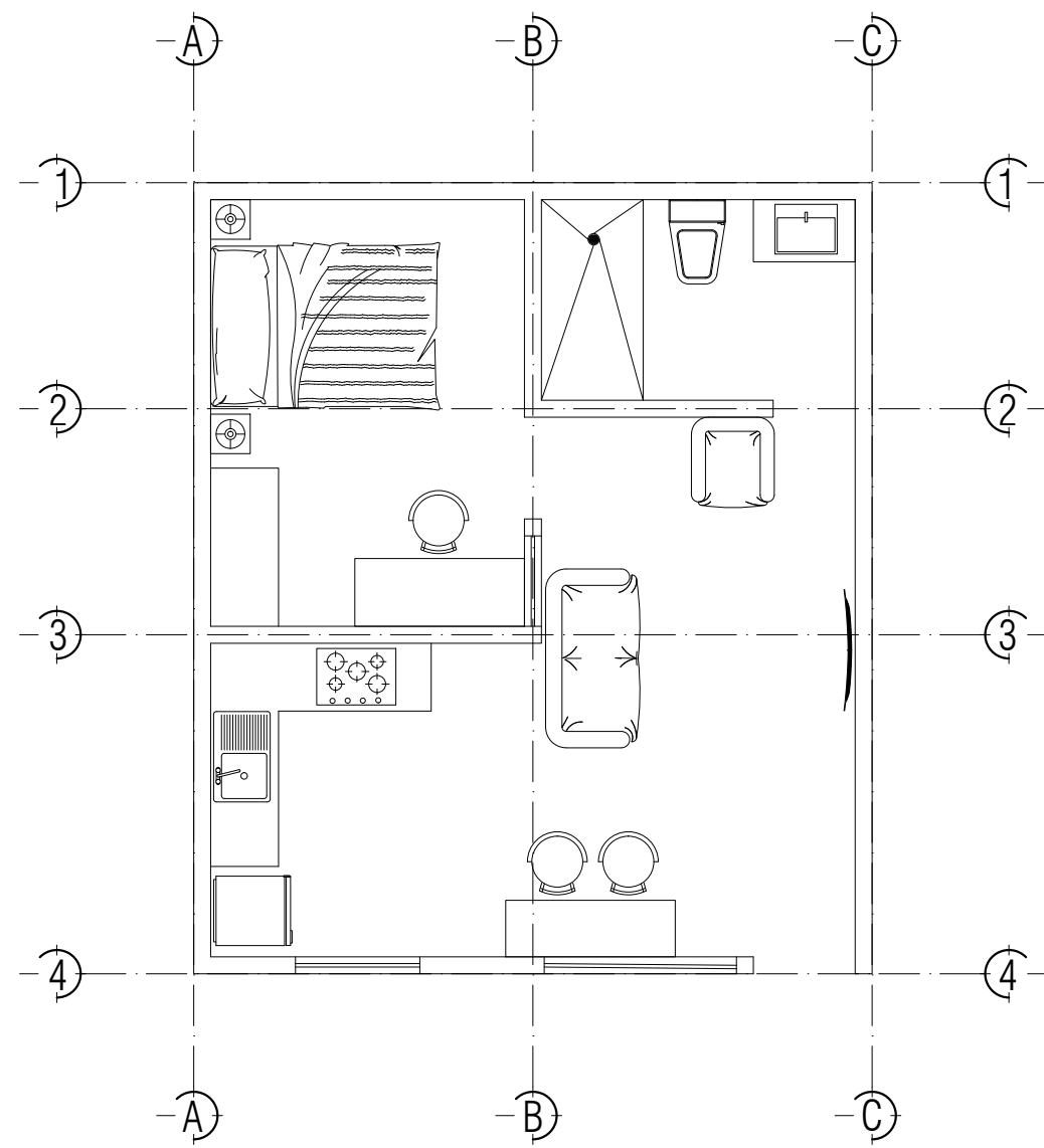
PLANTA ARQUITECTÓNICA
