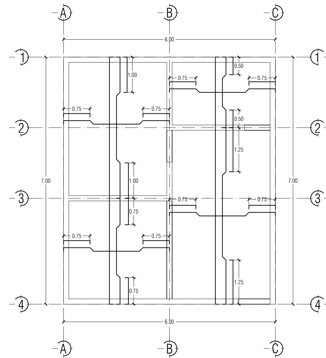
PLANTA ESTRUCTURAL
