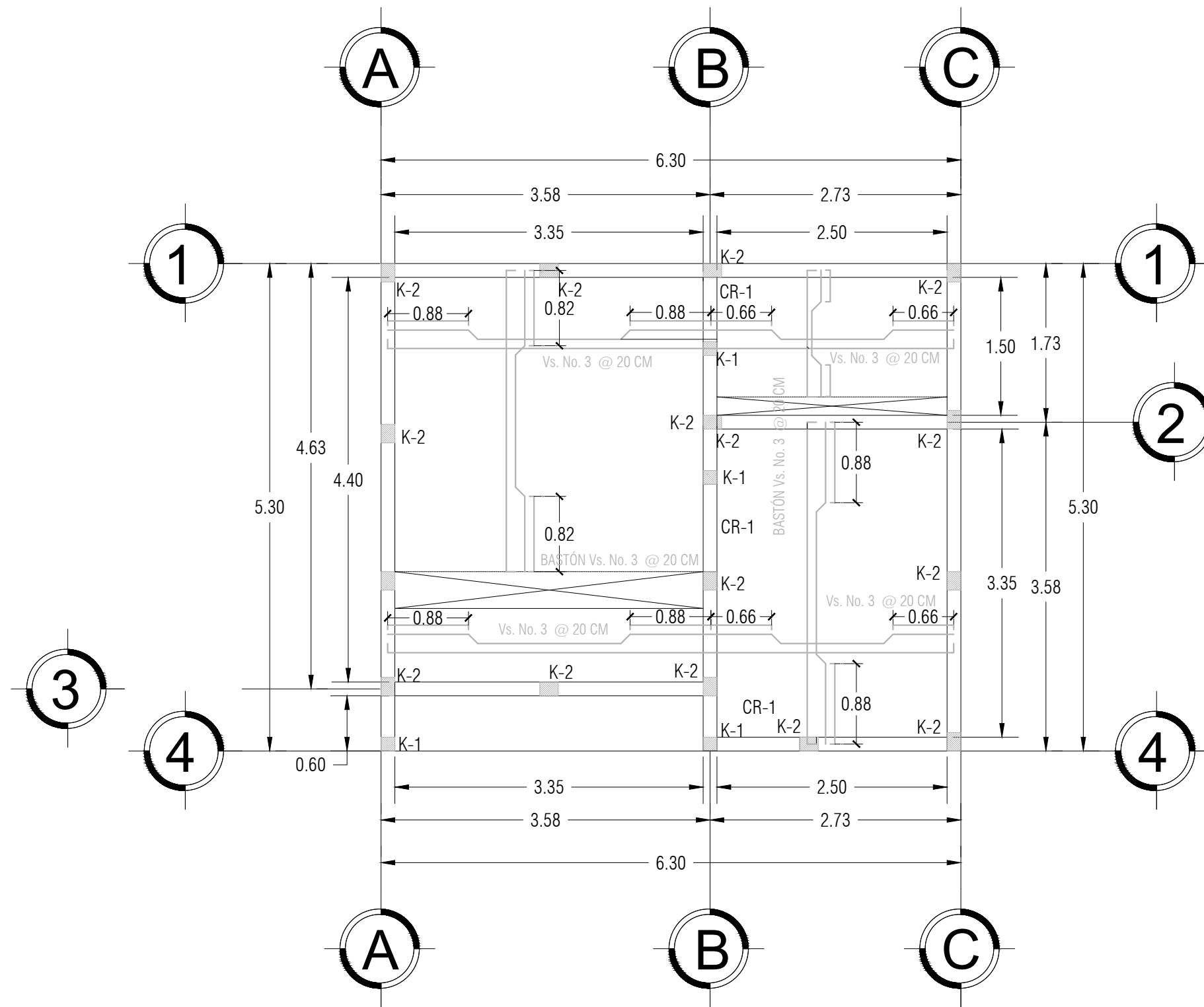
PLANTA ESTRUCTURAL 1:50
