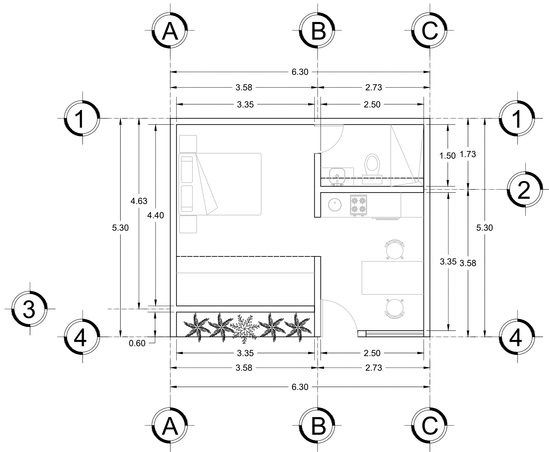
PLANTA ARQUITECTÓNICA 1:50
