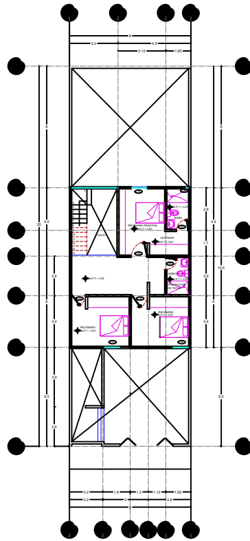
PLANTA ALTA ESC: 1:75
