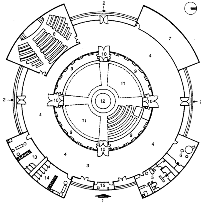
Planta general
