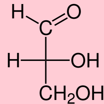
Triosas
