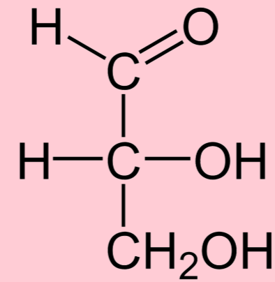
Aldosas
