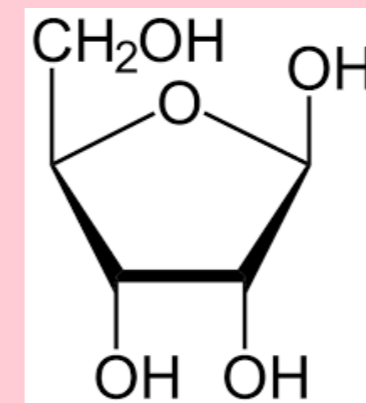
Pentosas
