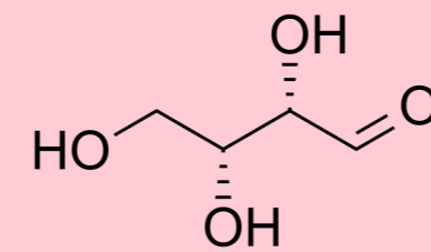
Tetrosas
