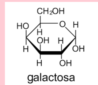
Hexosas
