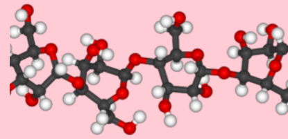
Polisacaridos
