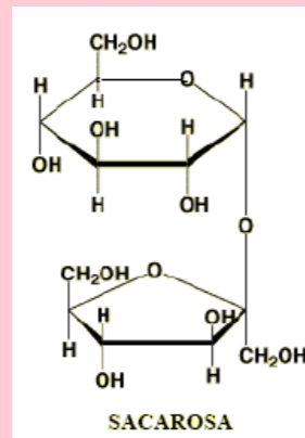
Disacáridos
