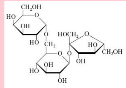
Oligosacaridos
