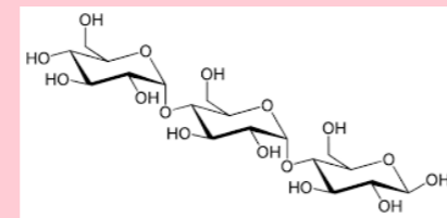
Trisacáridos
