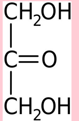
Cetosos
