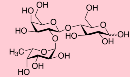
Monosacáridos
