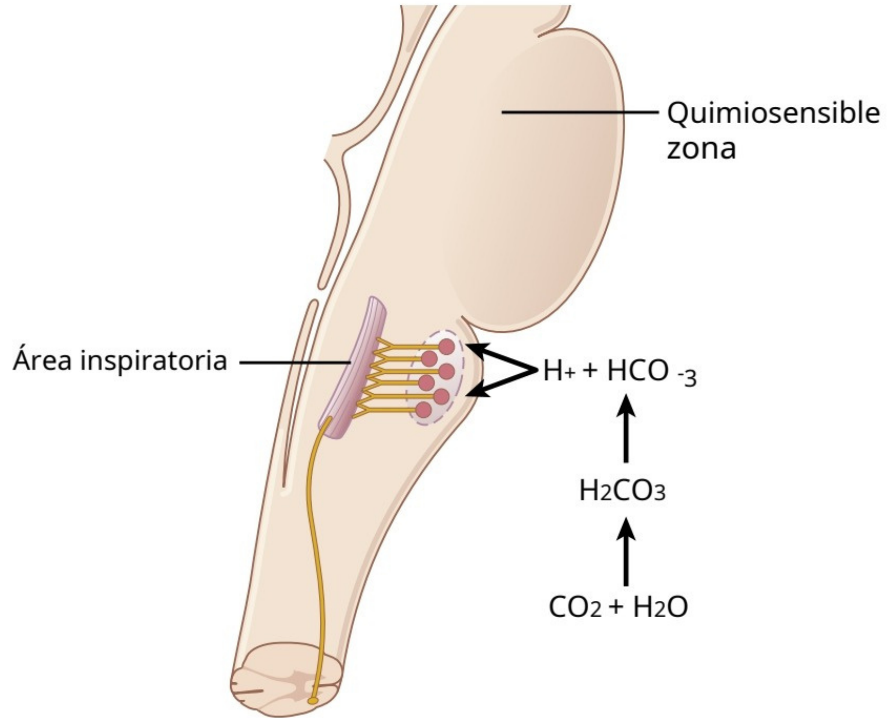
Figura 42-2. Estimulación de la inspiratorio del tronco encefálico área por señales del área quimiosensible localizada bilateralmente en la médula, situada sólo una fracción de milímetro por debajo de la superficie medular ventral. Tenga en cuenta también que H^+ estimula el área quimiosensible, pero el dióxido de carbono en el líquido da lugar a la mayor parte del H^+ .
