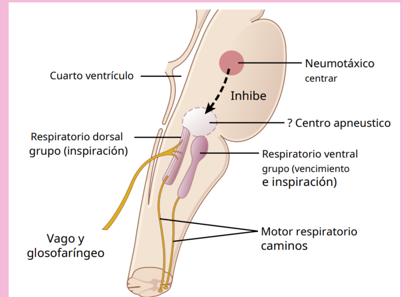
Figura 42-1. Organización del centro respiratorio.
