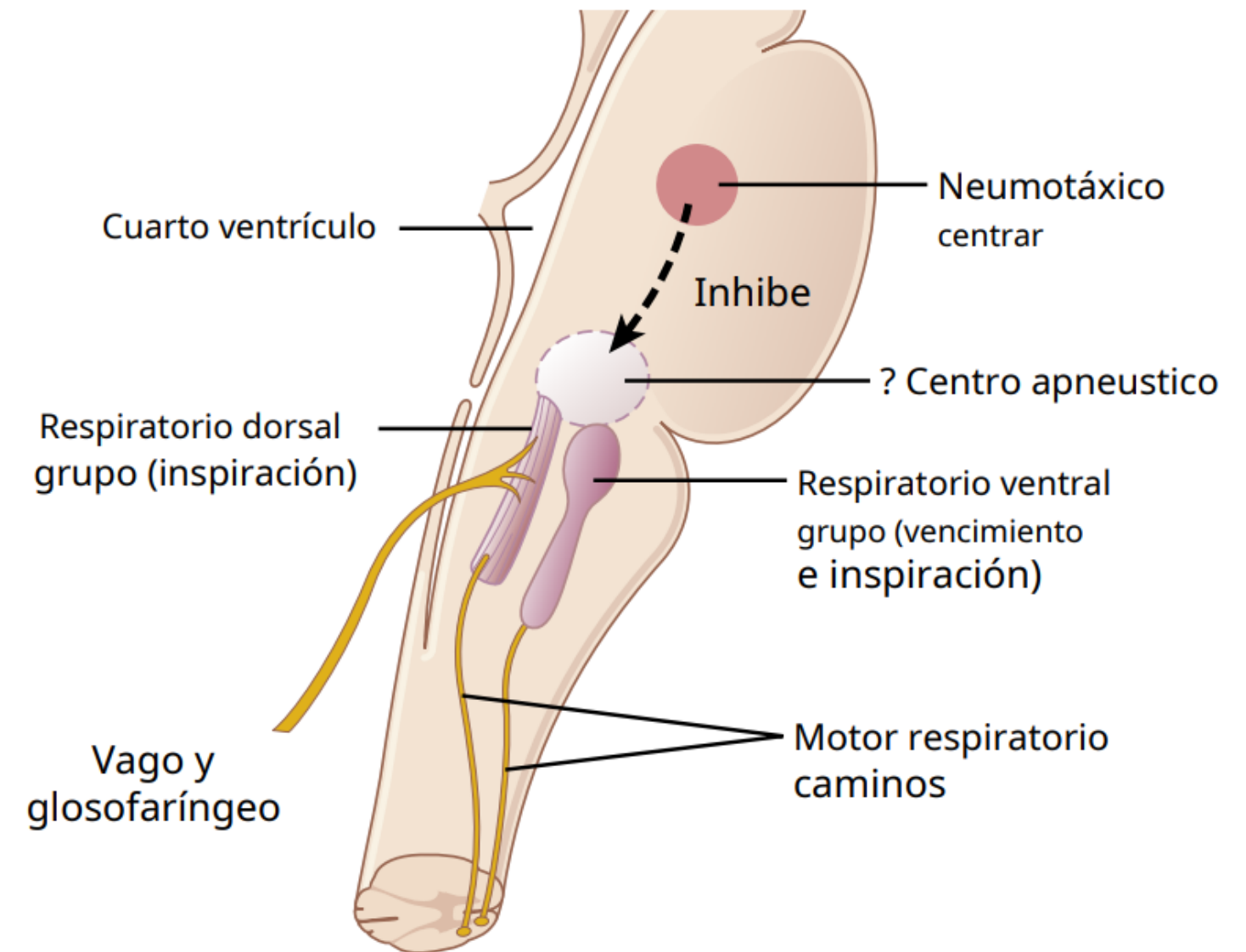
Figura 42-1. Organización del centro respiratorio.
