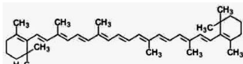
Figura 7. Fórmula del aceite de oliva.
