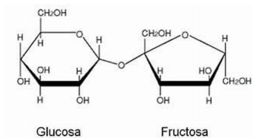
Figura 10. Fórmula de la sacarosa.
