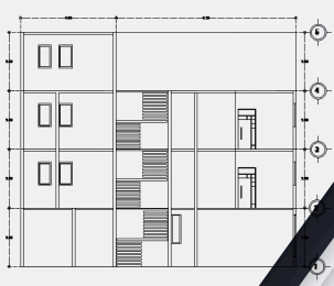
CORTE TRANSVERSAL
