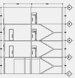
CORTE LONGITUDINAL
