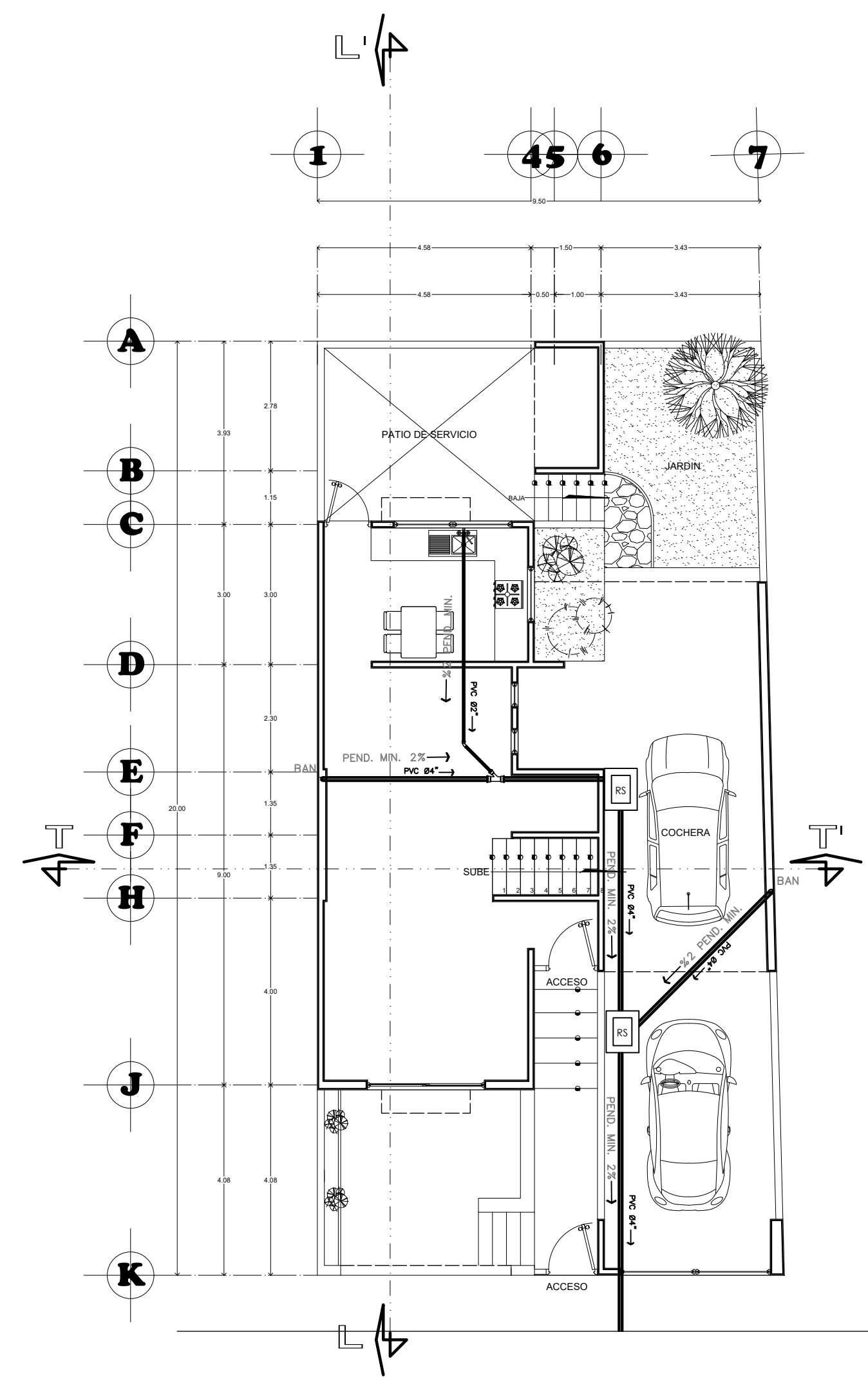
PLANTA BAJA ESCALA - 1:100
