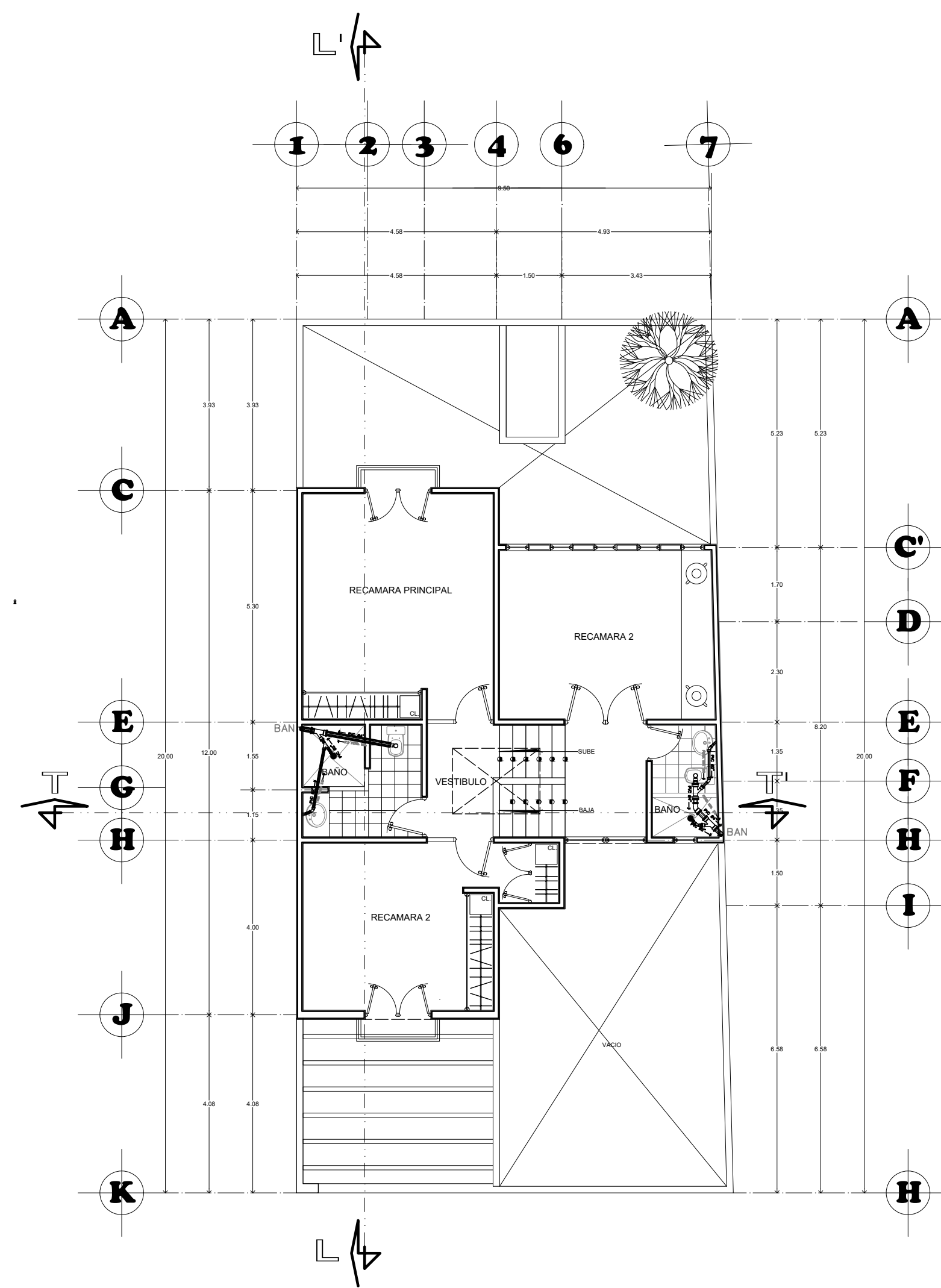
PLANTA ALTA ESCALA - 1:100
