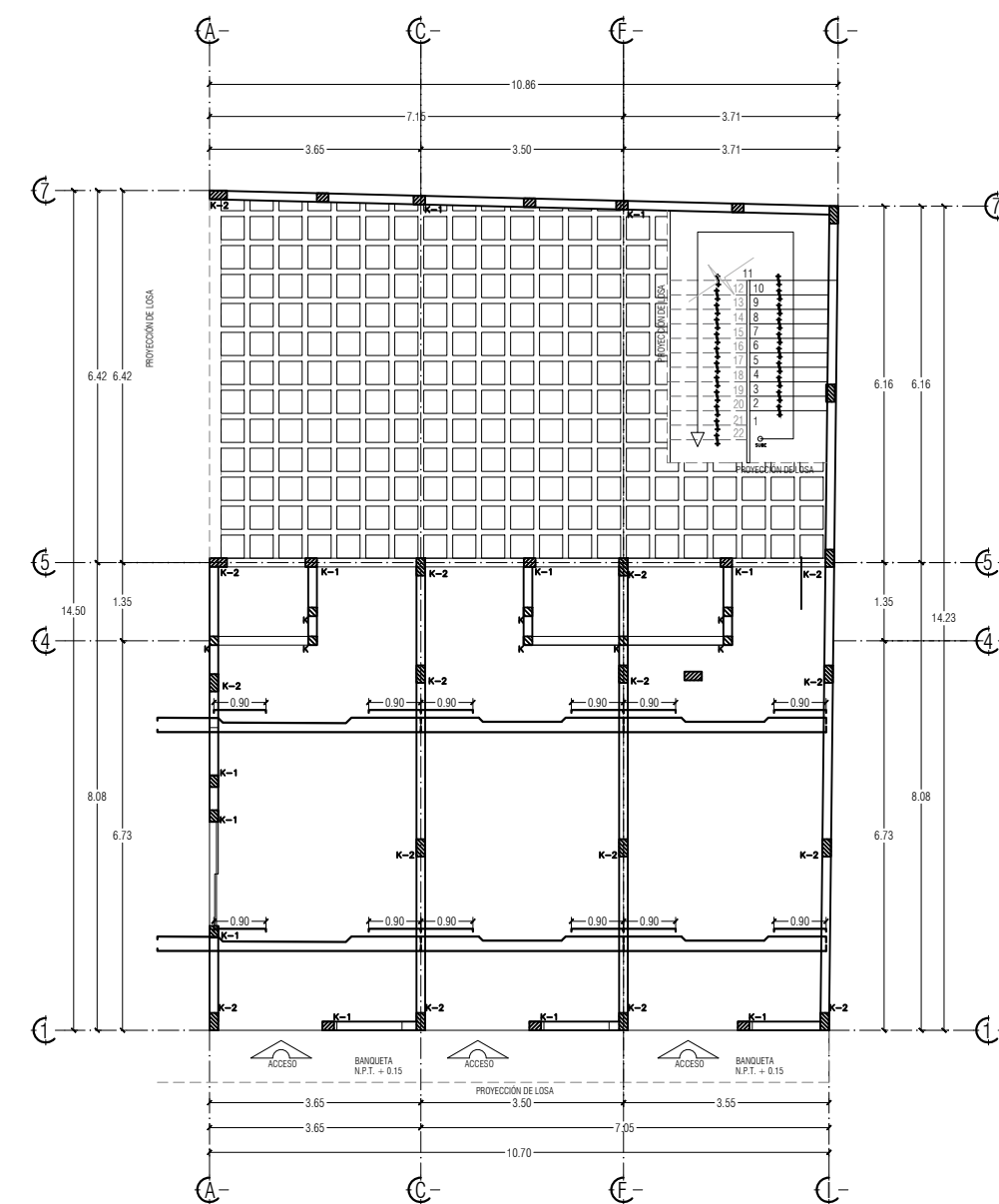
PLANTA BAJA ESC: 1/75
