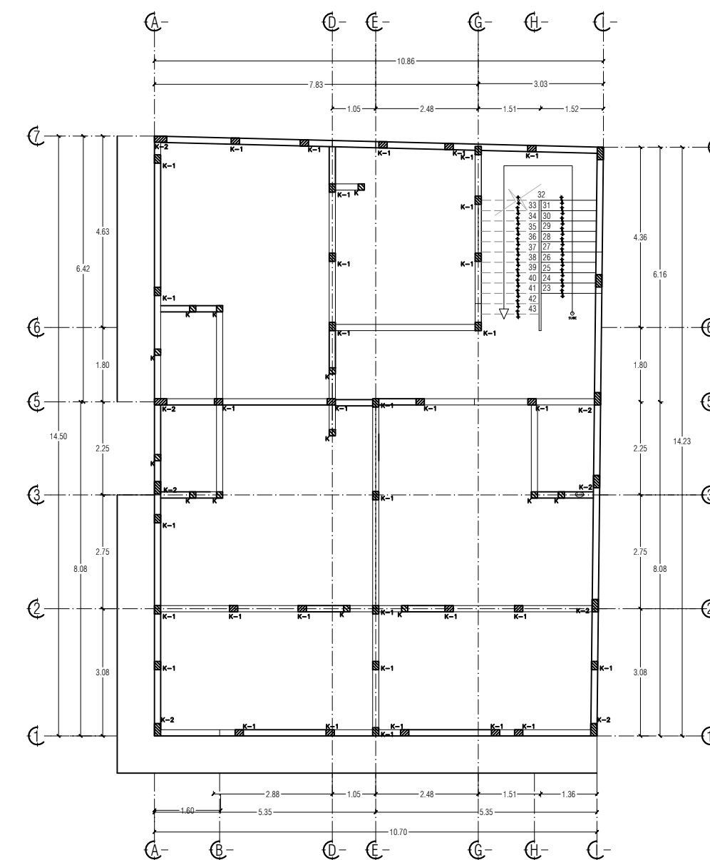
PLANTA ALTA ESC: 1/75
