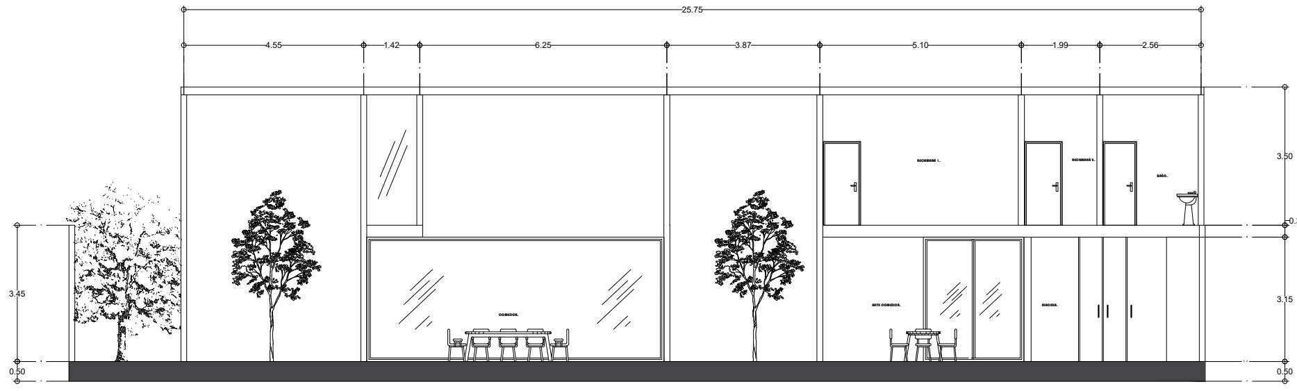
CORTE TRANSVERSAL.
