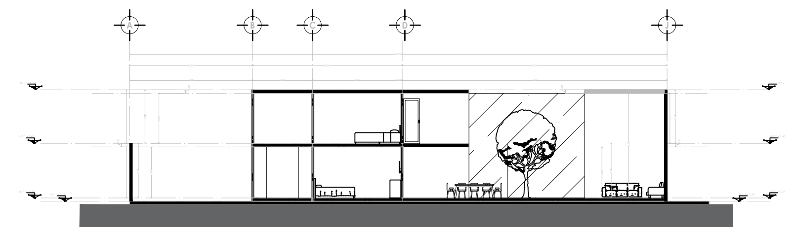
CORTE TRANSVERSAL B-B'
