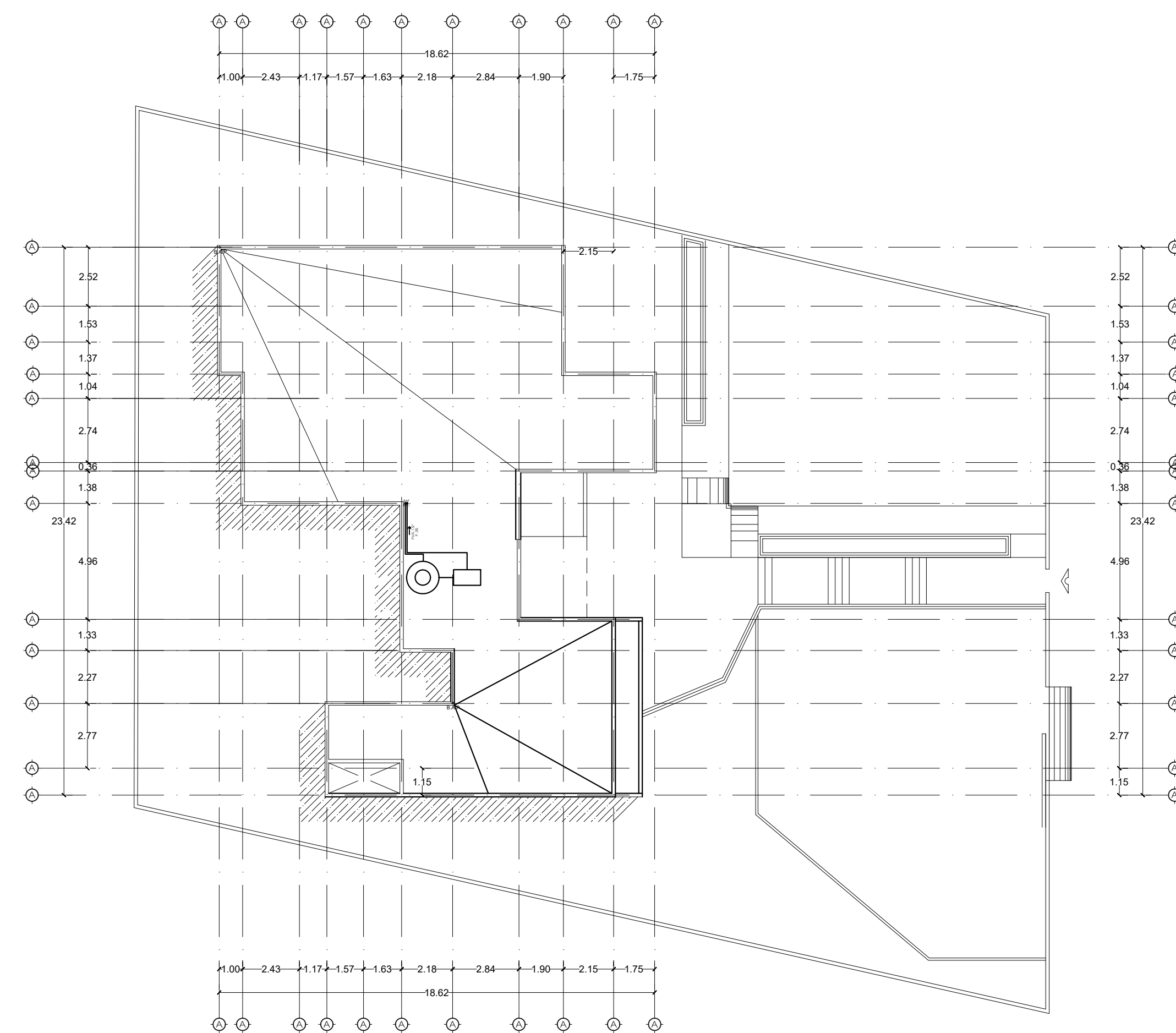
PLANTA ARQUITECTÓNICA DE CONJUNTO ESCALA 1:125
