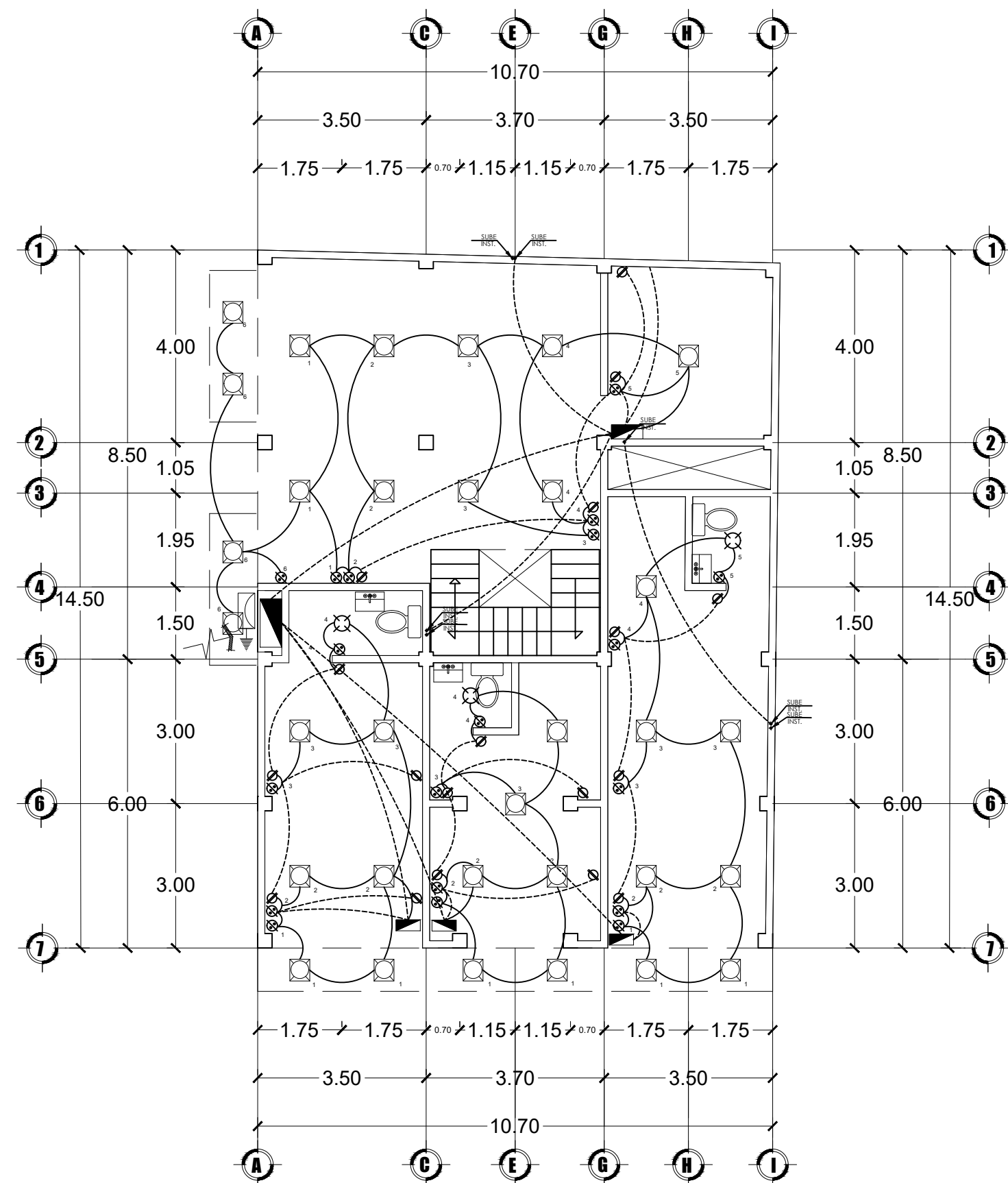
INSTALACIÓN ELÉCTRICA PLANTA BAJA
