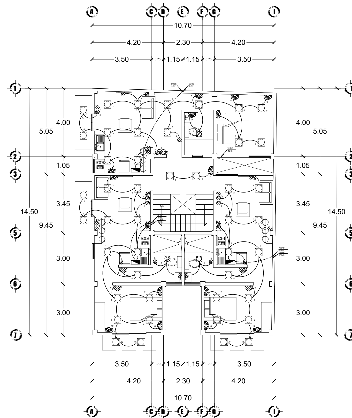
INSTALACIÓN ELÉCTRICA 1ER Y 2DO PISO
