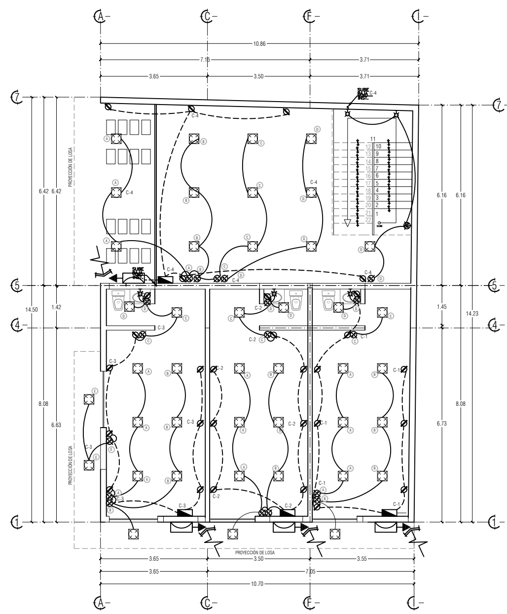
PLANTA BAJA ESC. 1:125
